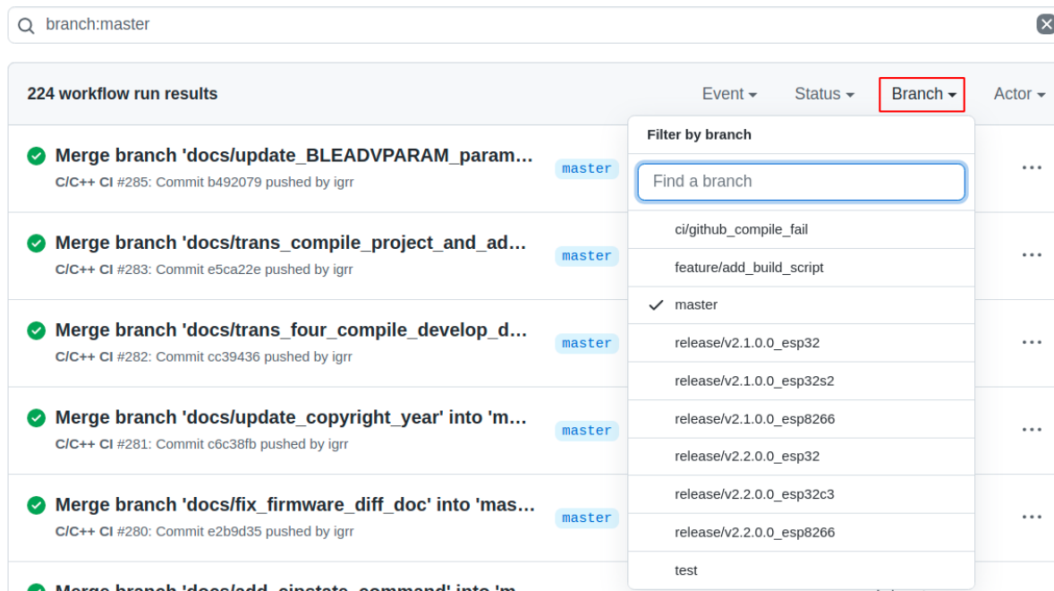
图 33: 点击 Branch
