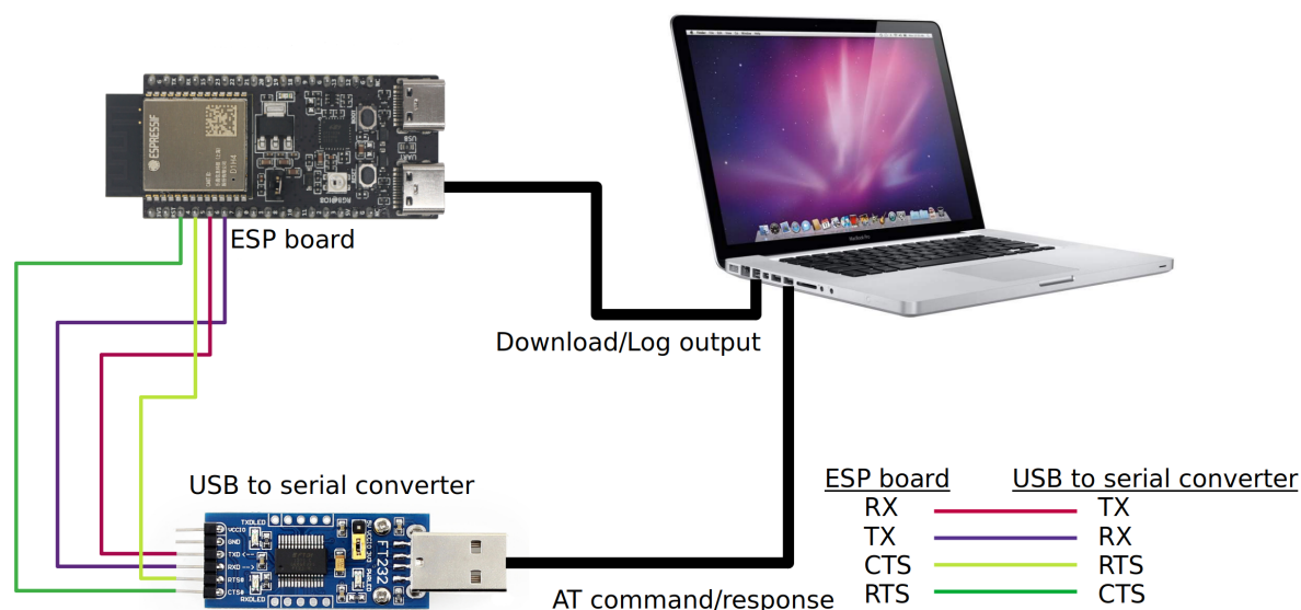
图 3: ESP32-C61-4MB 系列硬件连接示意图
