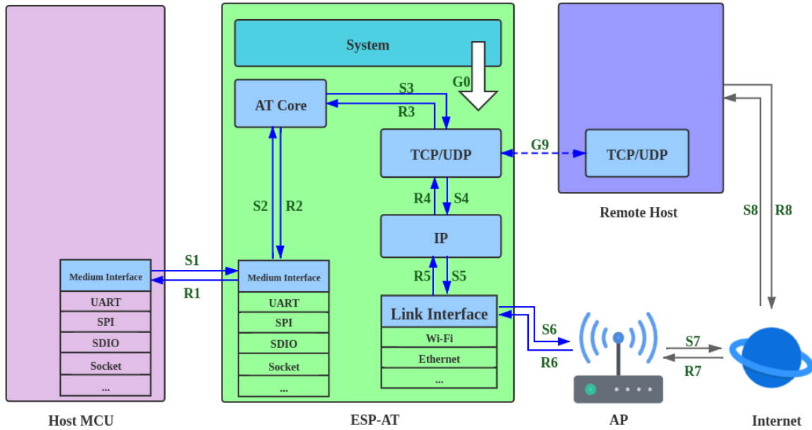
图 2: 吞吐数据流
