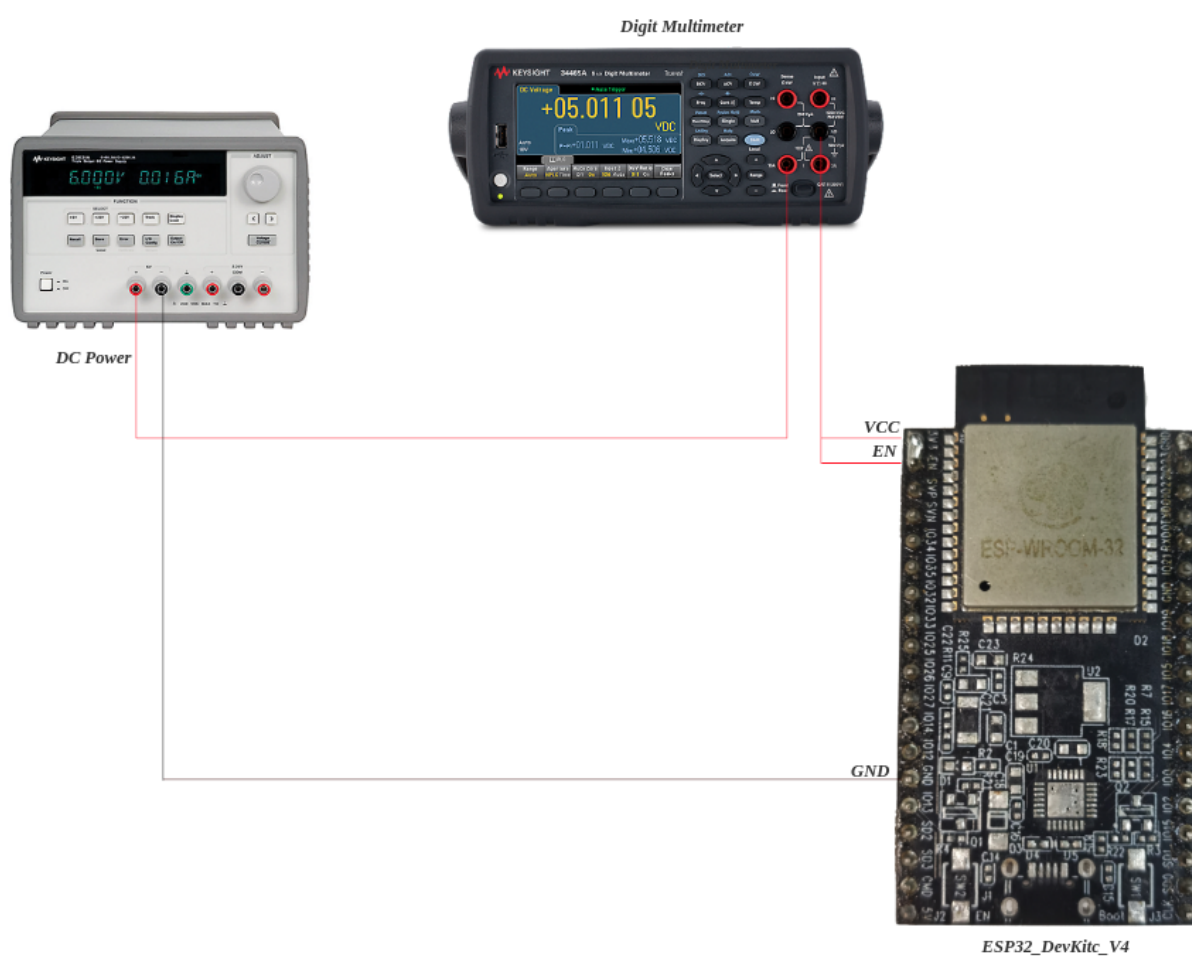
图 22: ESP32 硬件连接
