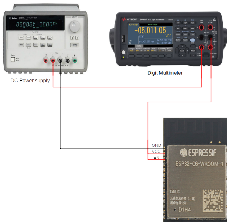
图 22: ESP32-C6 硬件连接
