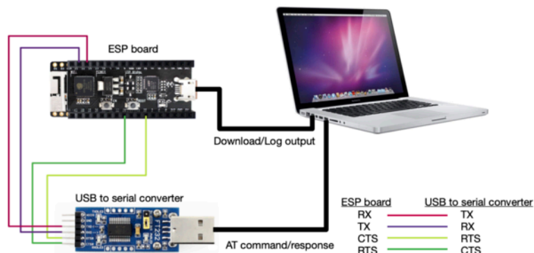
图 6: ESP32-PICO 系列硬件连接示意图
