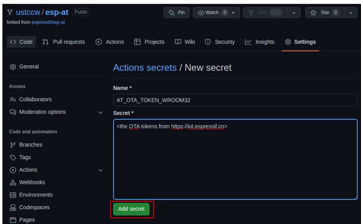
图 10: 创建密钥
