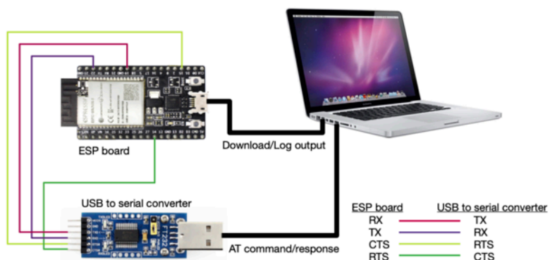
图 5: ESP32-WROVER 系列硬件连接示意图
