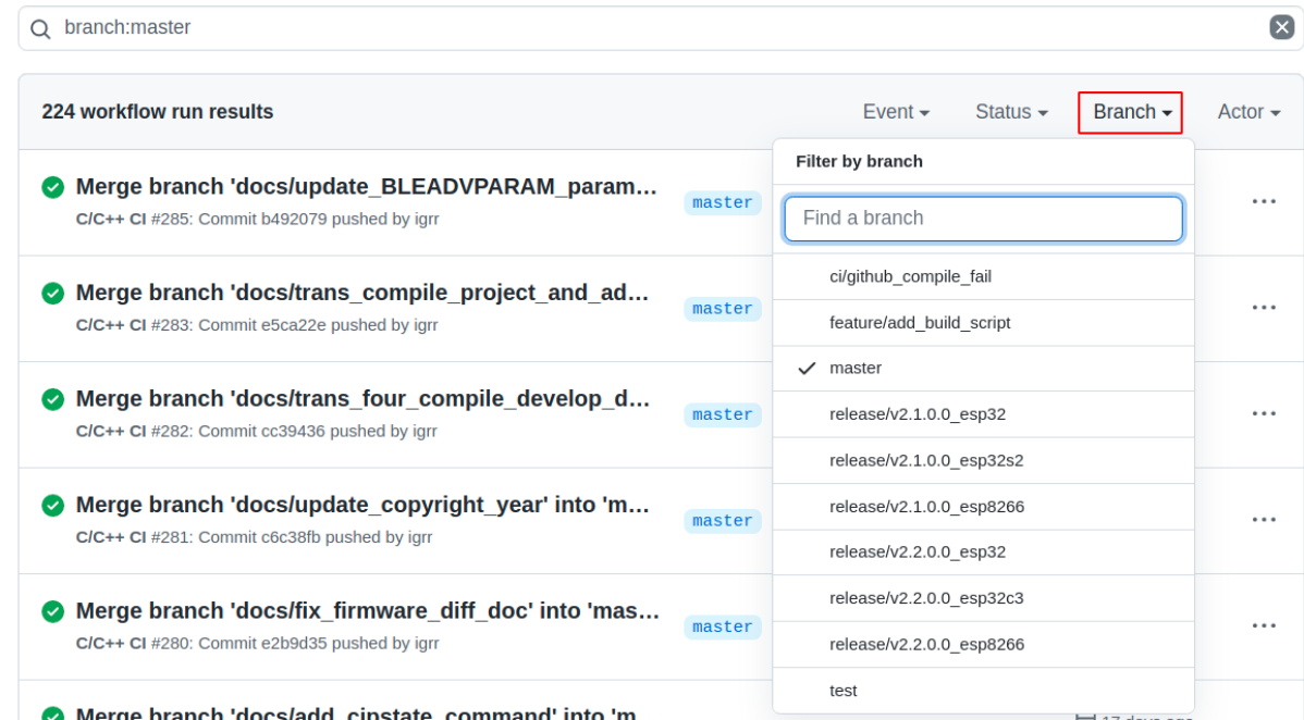
图 33: 点击 Branch
