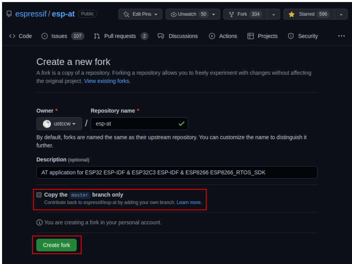
图 3: 创建 Fork
