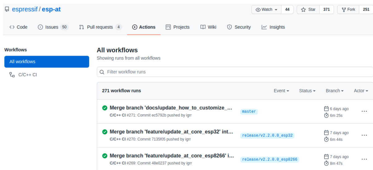
图 32: Actions 页面
