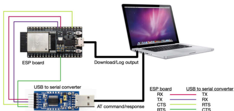
图 3: ESP32-WROOM-32 系列硬件连接示意图
