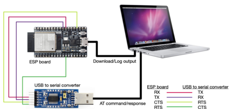
图 7: ESP32-SOLO 系列硬件连接示意图
