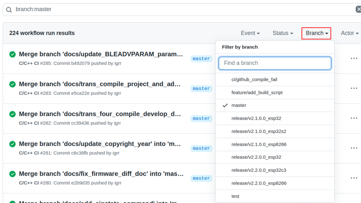
图 33: 点击 Branch
