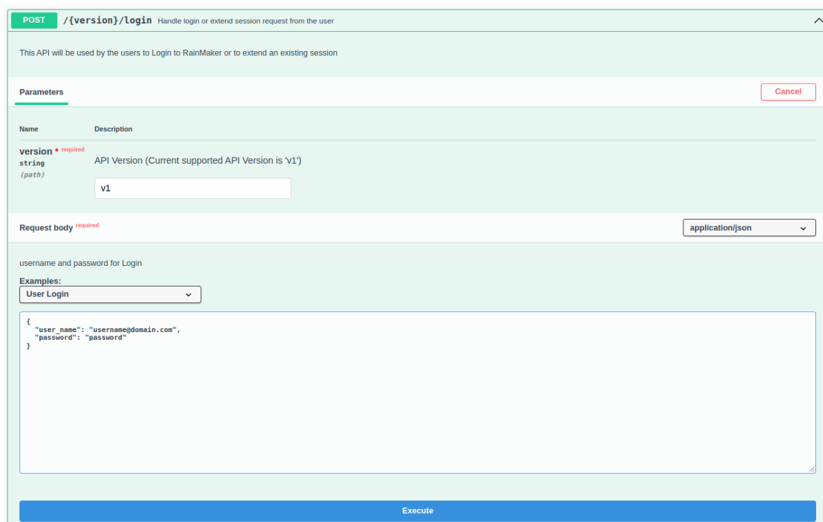
图 6: REST API 登陆
