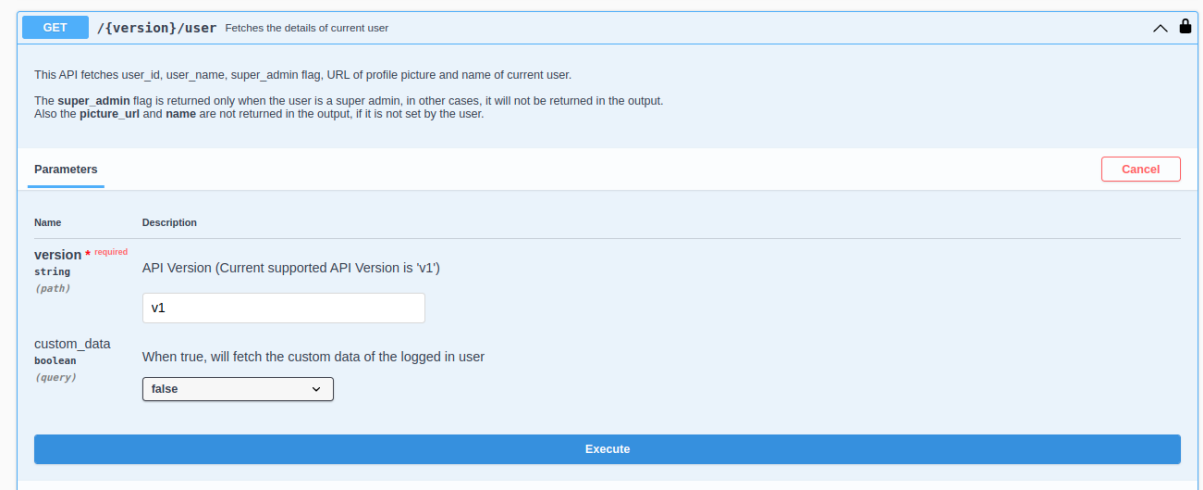
图 9: REST API 获取用户细节
