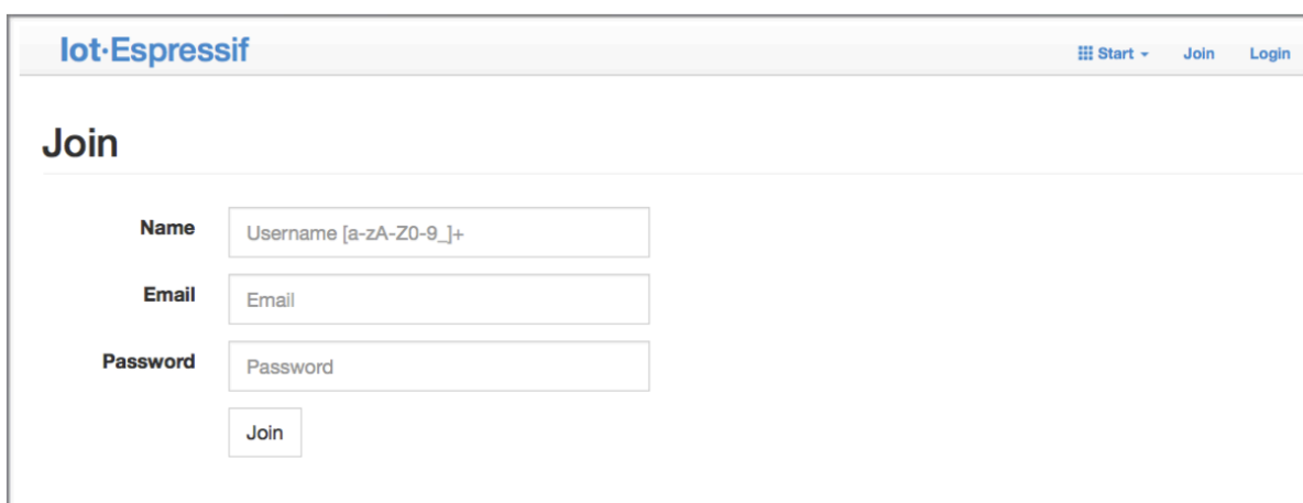
图 22: 加入 iot.espressif.cn
