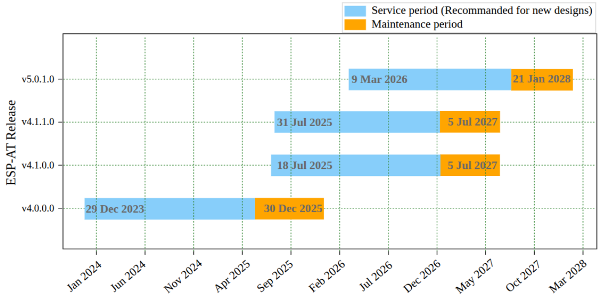
图 1: ESP-AT 版本支持期限
