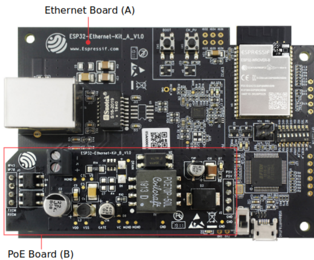
图 8: ESP32-Ethernet-Kit V1.0
