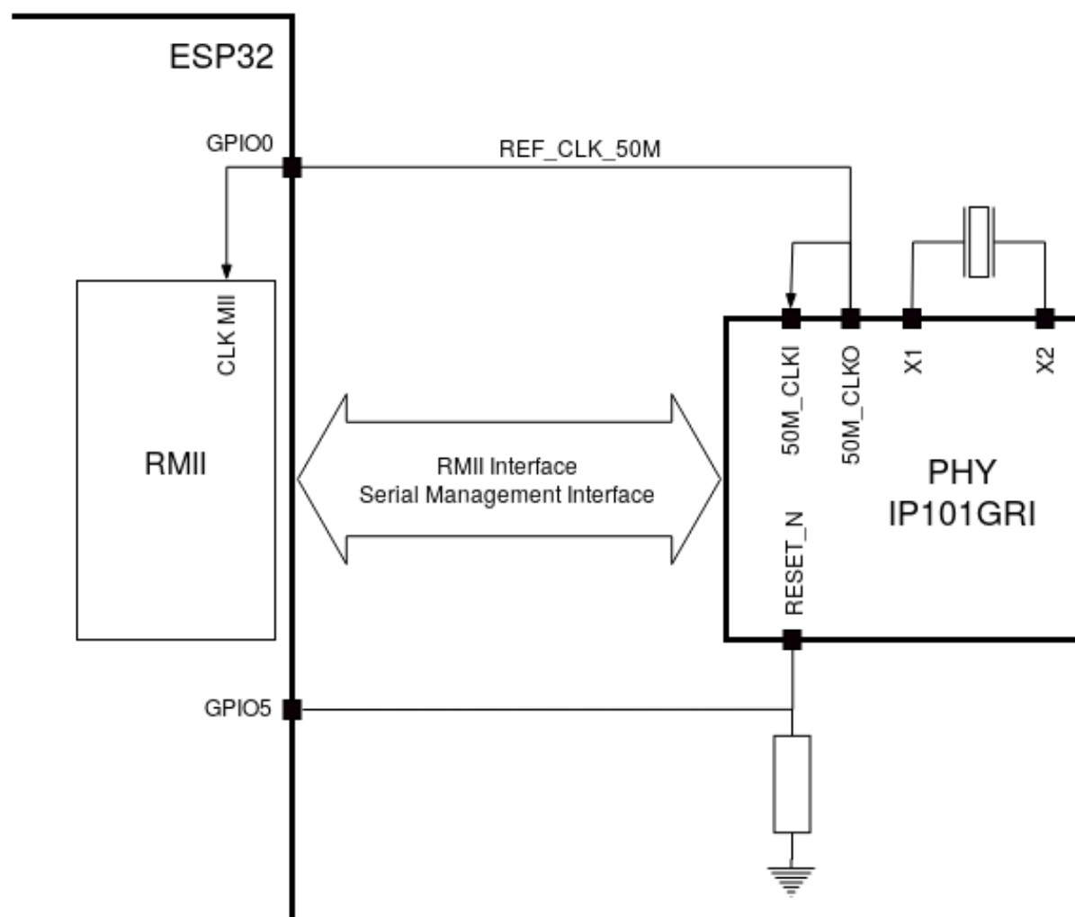
图 16: PHY 侧提供 RMI 时钟 (点击放大)
