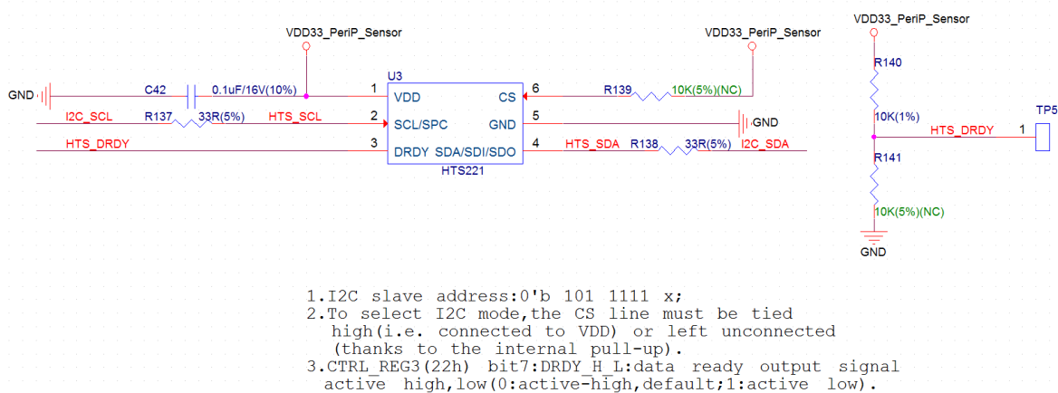
图 22: 温湿度传感器电路原理图
