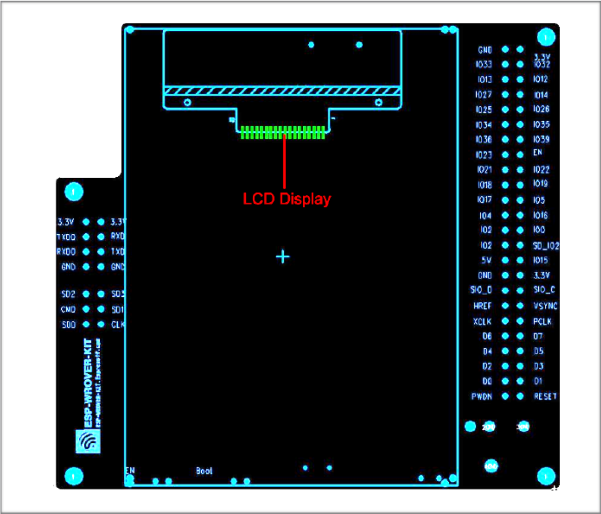
图 30: ESP-WROVER-KIT 开发板布局-仰视图
