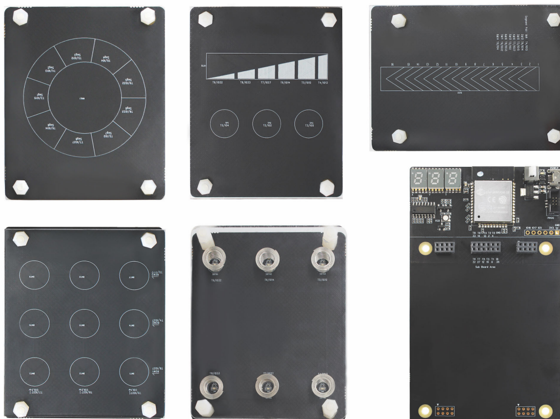
图 1: ESP32-Sense-Kit
