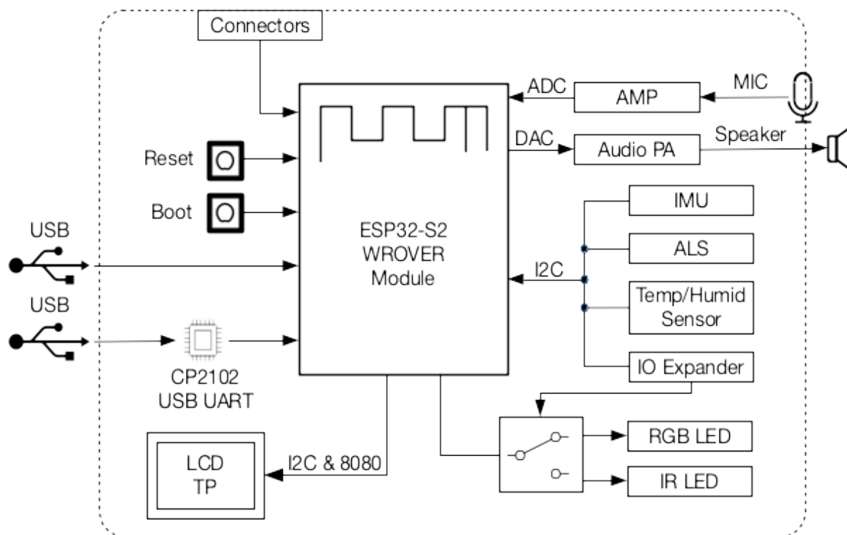
图 4: ESP32-S2-HMI-DevKit-1 功能框图
