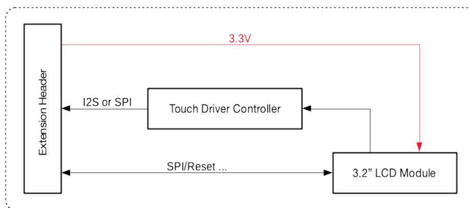
图 16: ESP-LyraP-LCD32 功能框图
