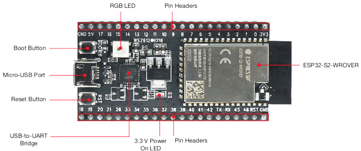
图 2: ESP32-S2-Saola-1 - 正面
