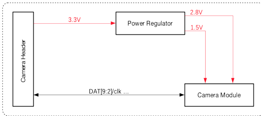
图 13: ESP-LyraP-CAM 功能框图
