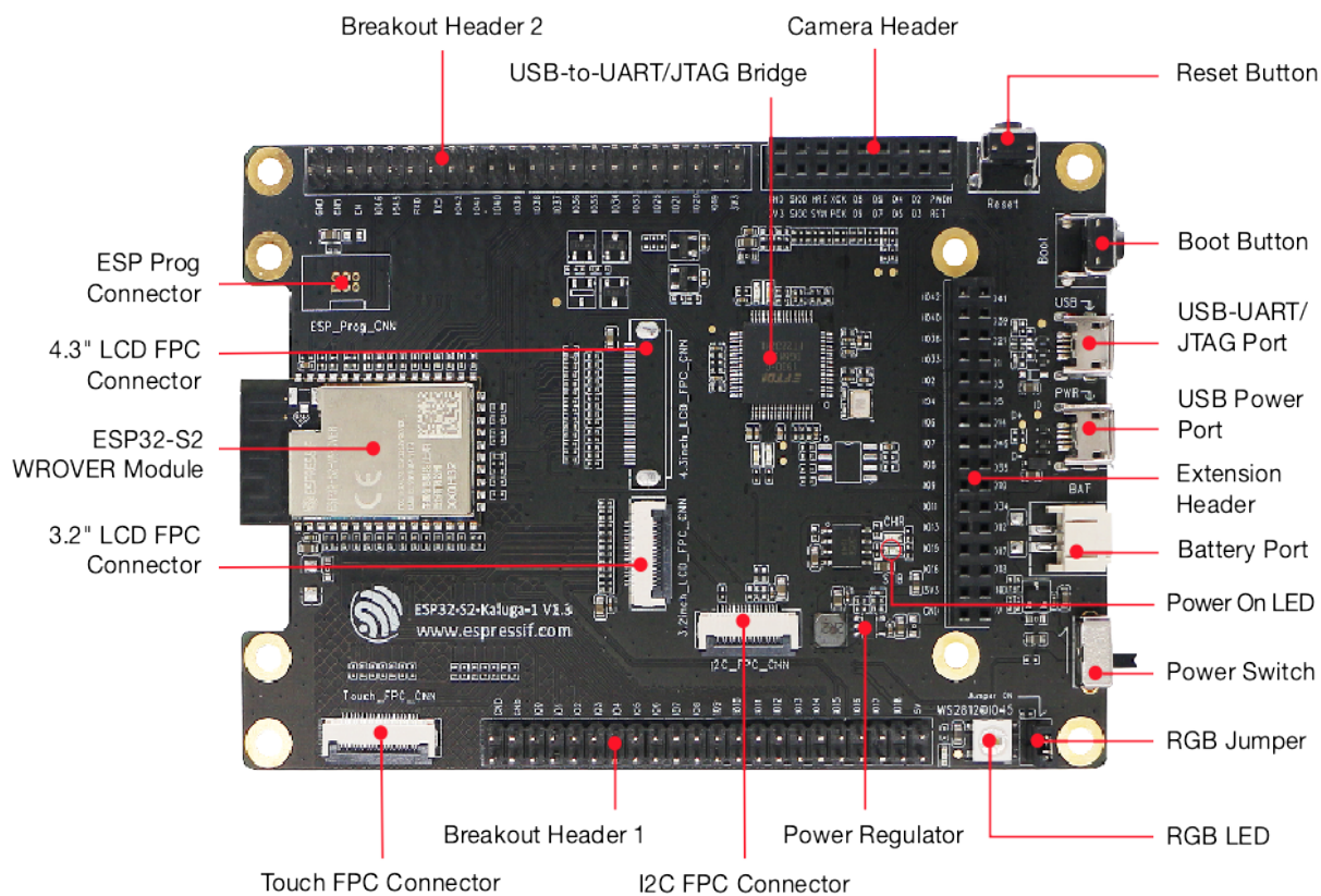
图 3: ESP32-S2-Kaluga-1 - 正面 (点击放大)
