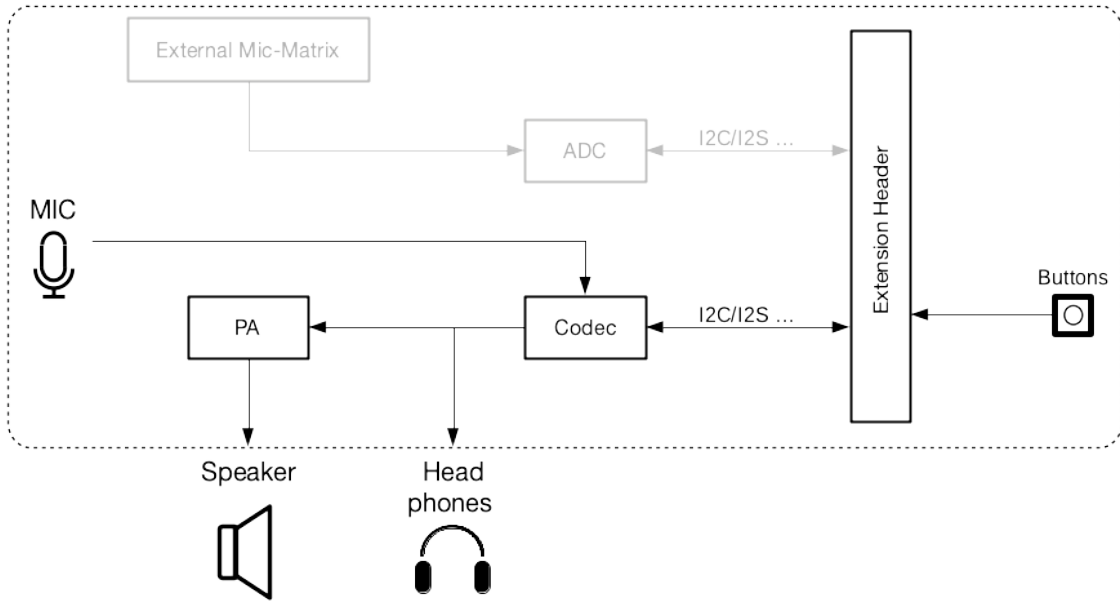
图 22: ESP-LyraT-8311A 功能框图
