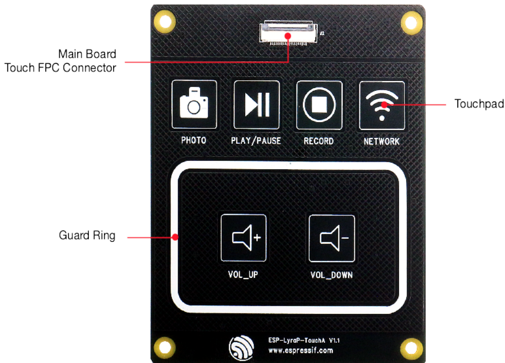
图 18: ESP-LyraP-TouchA
