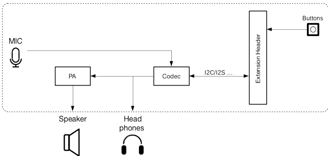
图 32: ESP-LyraT-8311A 功能框图
