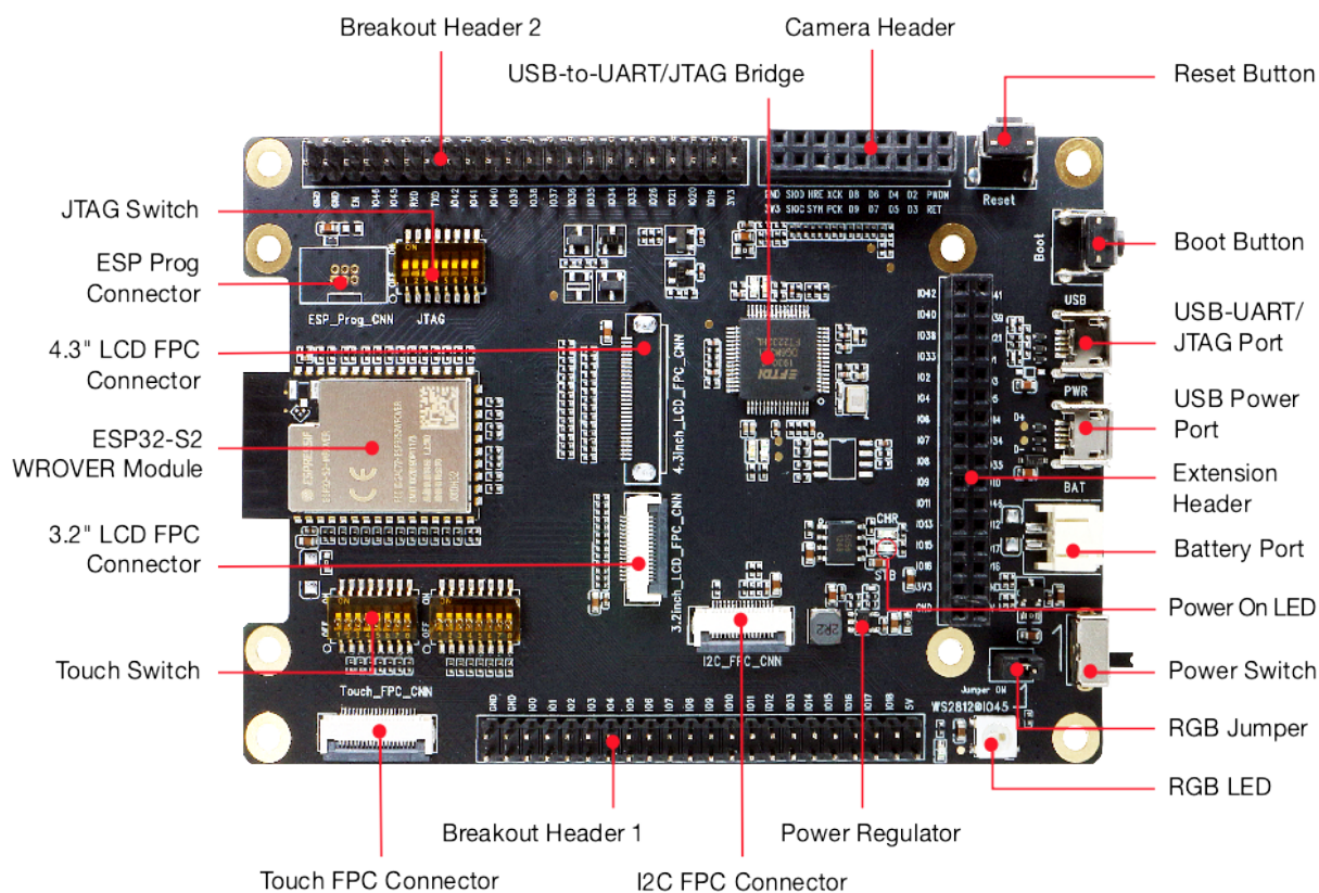
图 9: ESP32-S2-Kaluga-1 - 正面 (点击放大)
