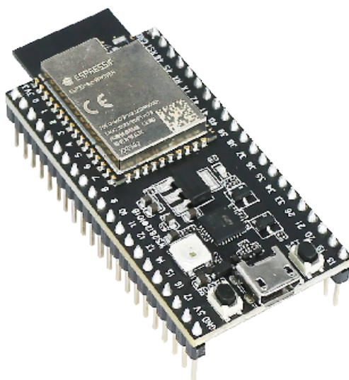
图 1: ESP32-S2-Saola-1
