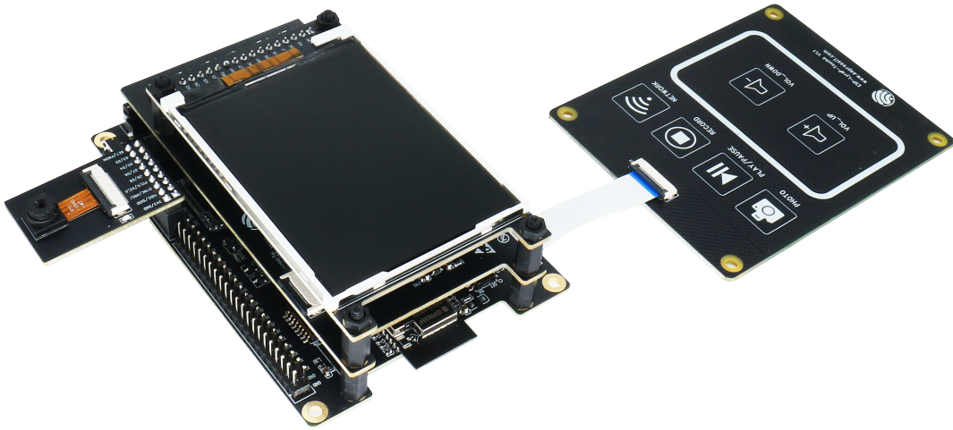
图 1: ESP32-S2-Kaluga-1-Kit 概述 (点击放大)
