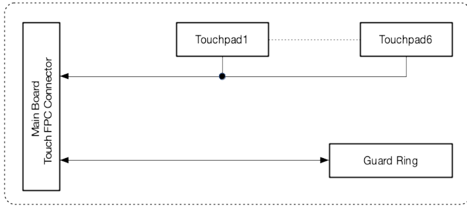
图 19: ESP-LyraP-TouchA-v1.1 功能框图
