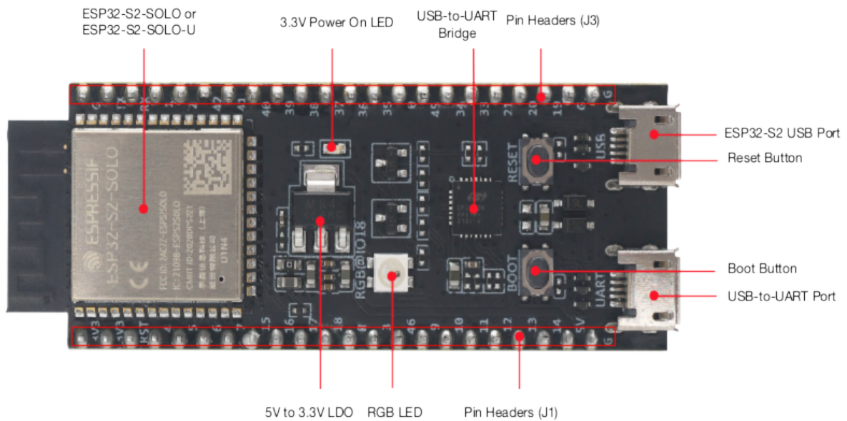
图 2: ESP32-S2-DevKitC-1 - 正面
