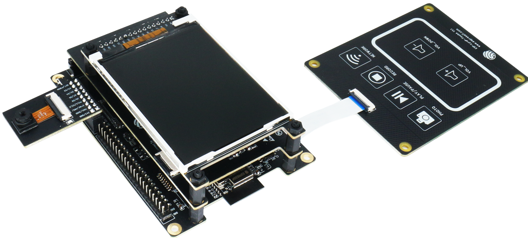
图 7: ESP32-S2-Kaluga-1-Kit 概述 (点击放大)
