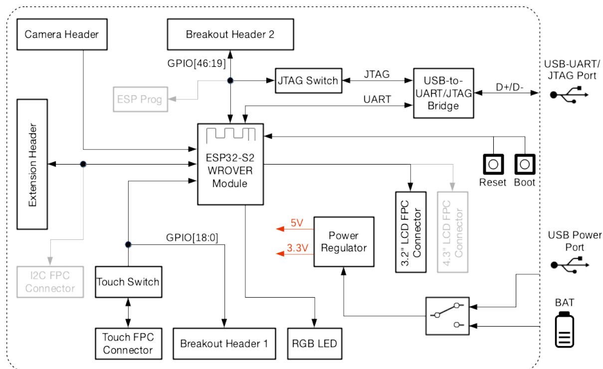
图 6: ESP32-S2-Kaluga-1 功能框图
