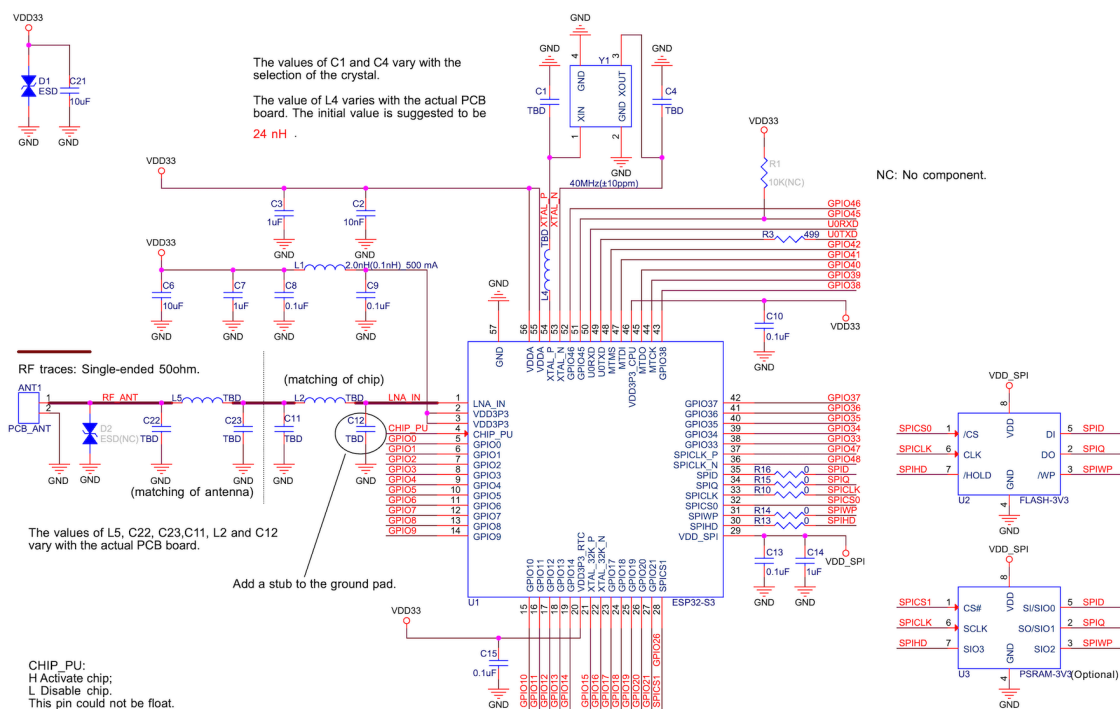
图 1: ESP32-S3 系列芯片参考设计原理图
