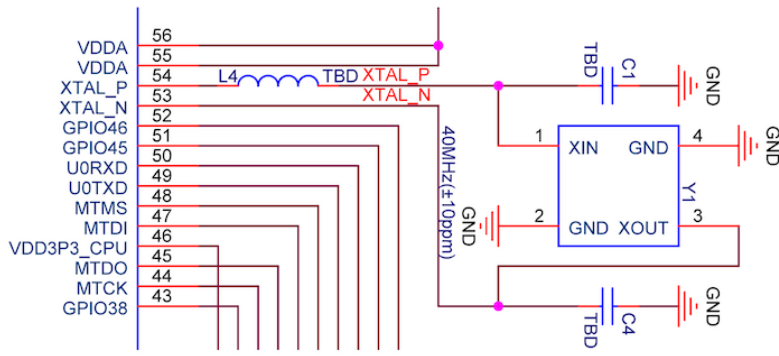
图 5: ESP32-S3 系列芯片无源晶振电路图
