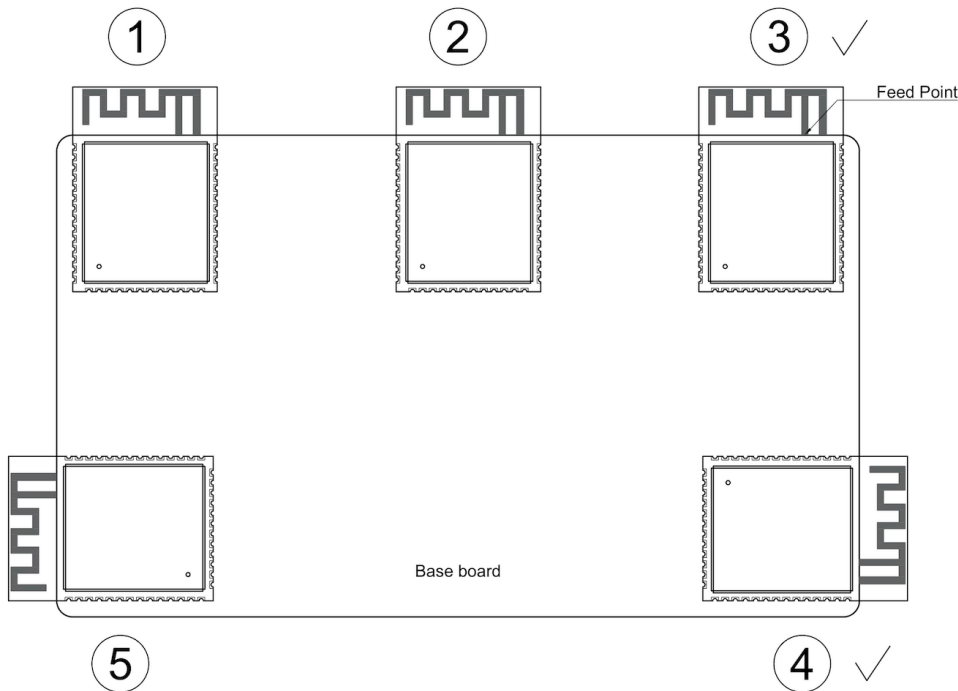
图 24: ESP32-S3 系列模组 (天线馈点在右侧) 在底板上的位置示意图
