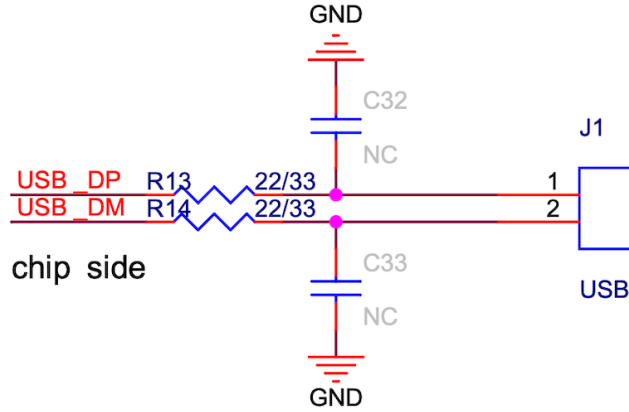
图 10: ESP32-S3 系列芯片 USB RC 电路图
