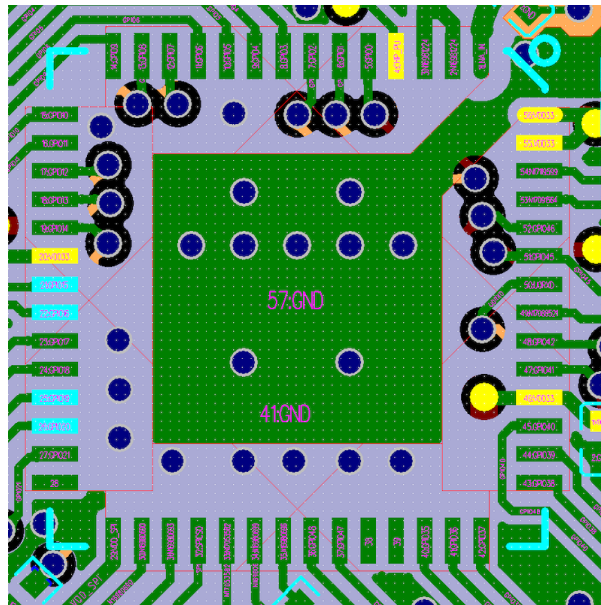
图 13: ESP32-S3 系列芯片底部 EPAD 设计
