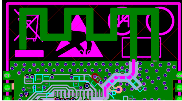
图 17: ESP32-S3 系列芯片四层板射频部分版图设计
