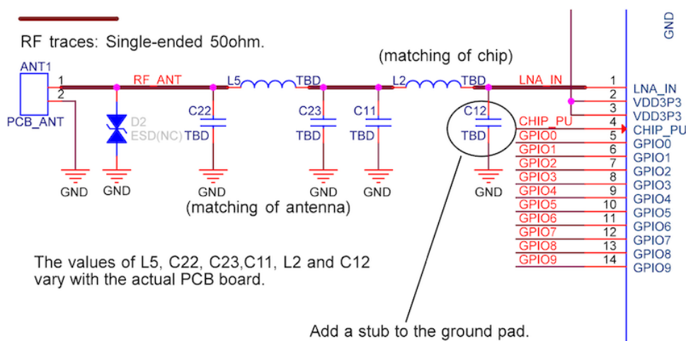
图 7: ESP32-S3 系列芯片射频匹配电路图
