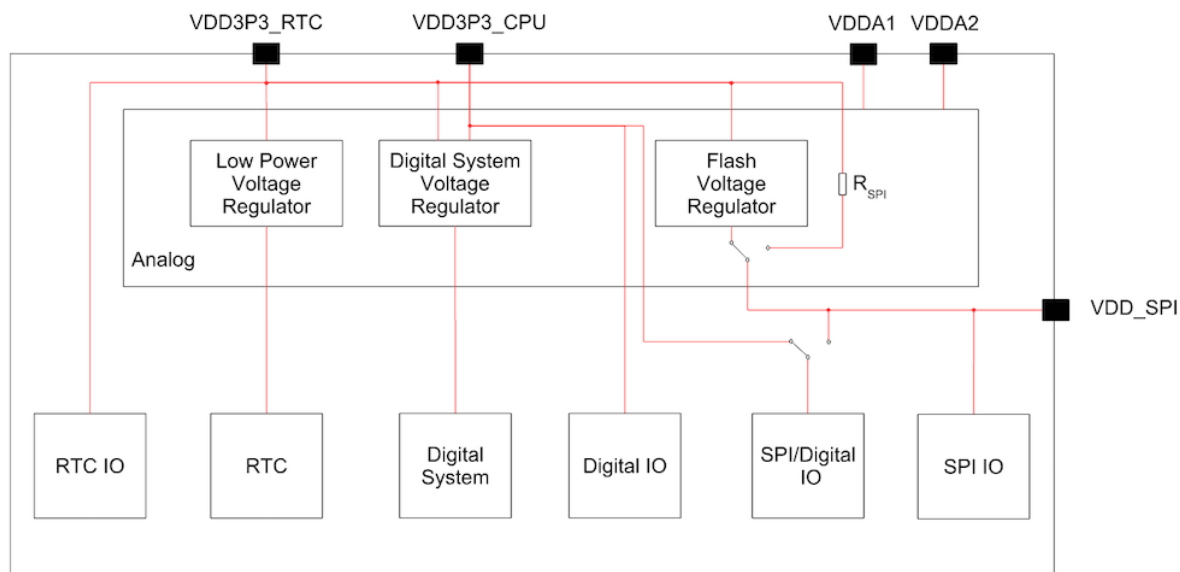
图 3: ESP32-S3 系列芯片电源管理图
