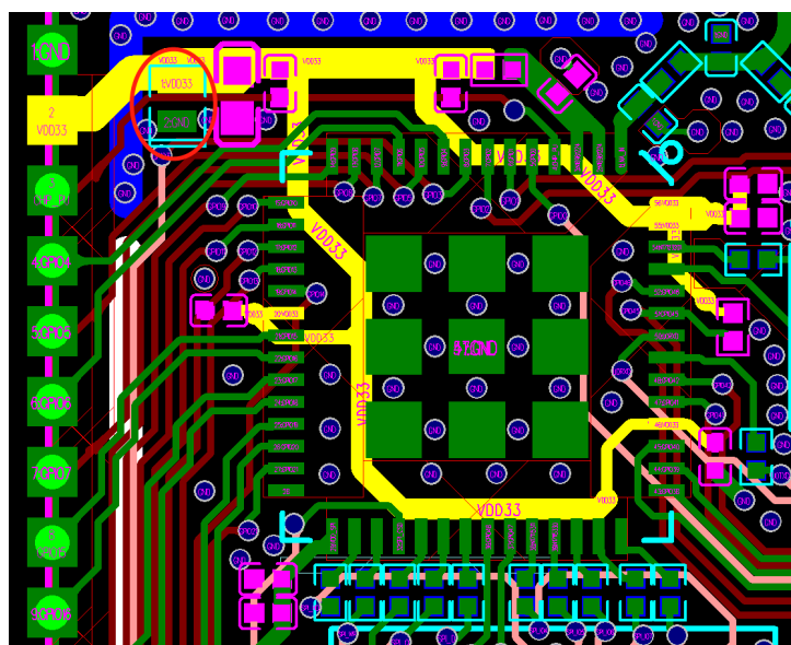
图 12: ESP32-S3 系列芯片四层板电源设计
