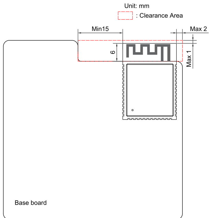
图 26: ESP32-S3 天线区域净空示意图
