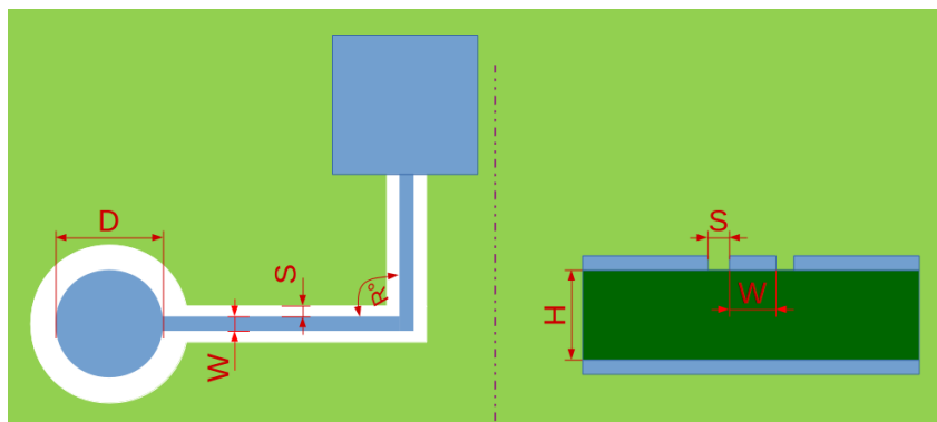
图 29: ESP32-S3 传感器布局布线
