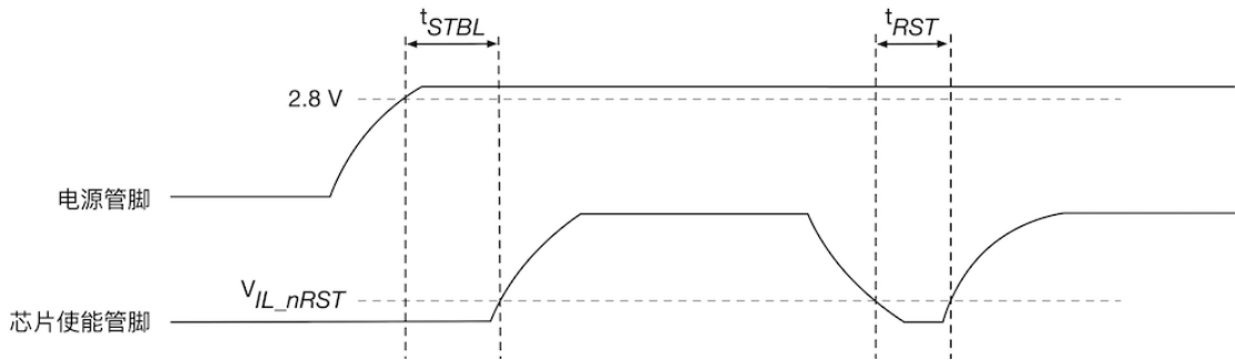
图 4: ESP32-S3 系列芯片上电和复位时序图
