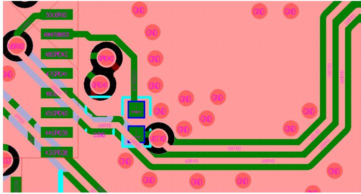
图 23: ESP32-S3 系列芯片 UART 版图设计
