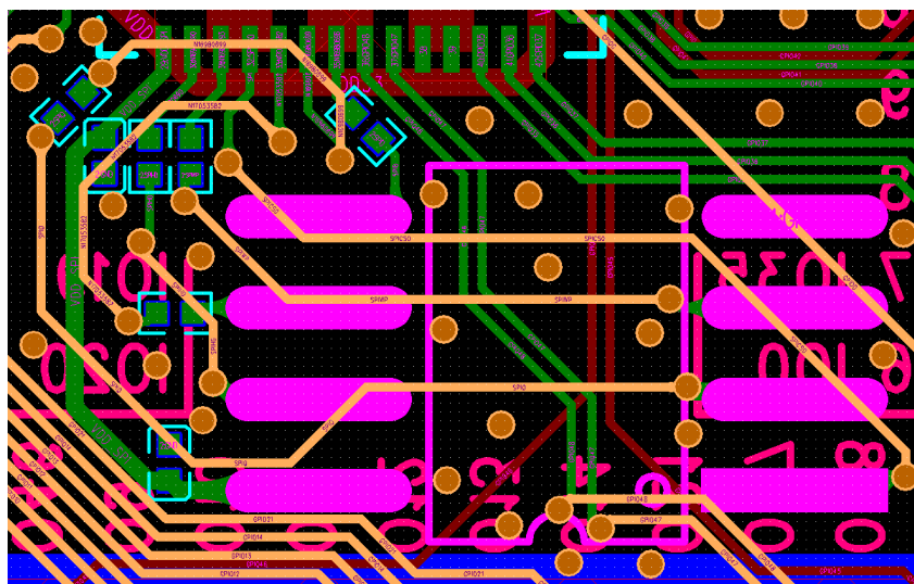
图 21: ESP32-S3 系列芯片 Quad SPI Flash 版图设计
