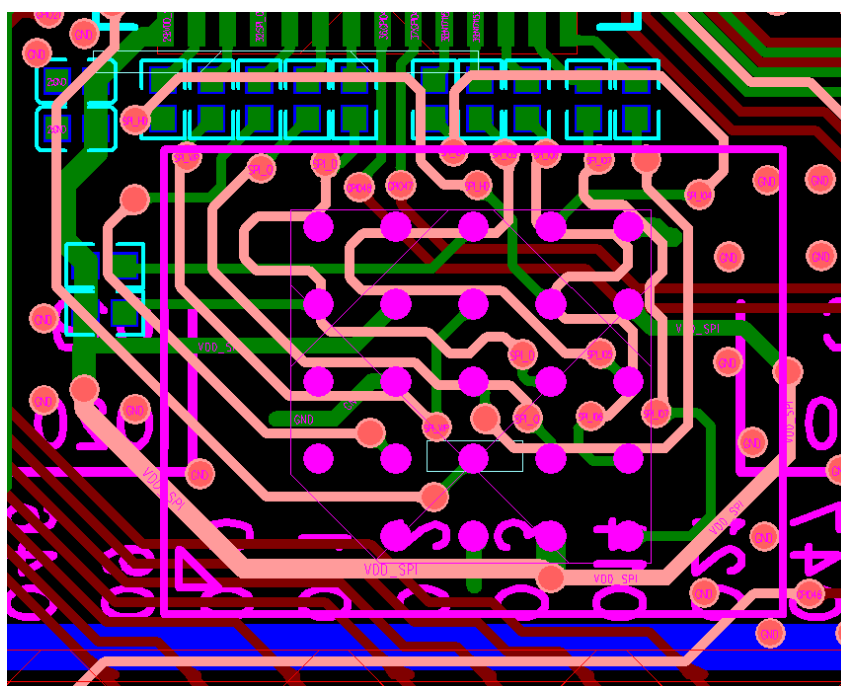
图 22: ESP32-S3 系列芯片 Octal SPI Flash 版图设计
