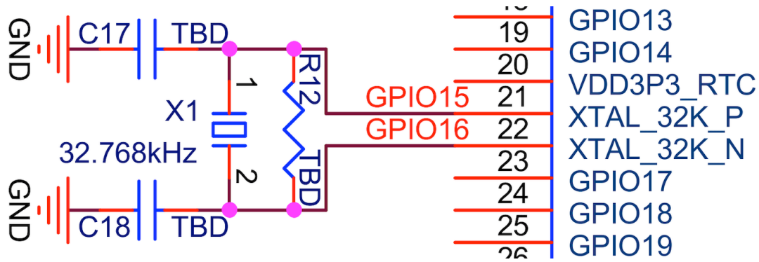
图 6: ESP32-S3 系列芯片外置 32.768 kHz 无源晶振电路图
