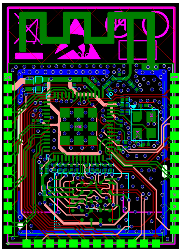
图 11: ESP32-S3 模组版图参考设计
