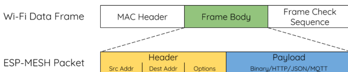
Fig. 56: ESP-WIFI-MESH Packet
