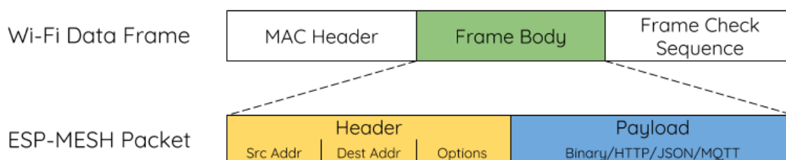
Fig. 55: ESP-WIFI-MESH Packet
