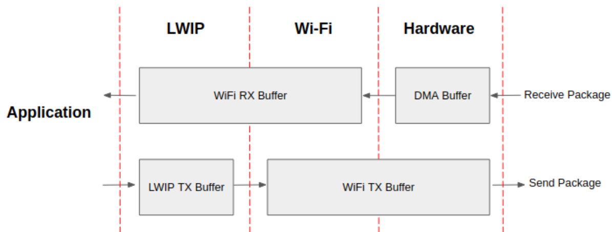
Fig. 54: ESP32-C2 datapath
