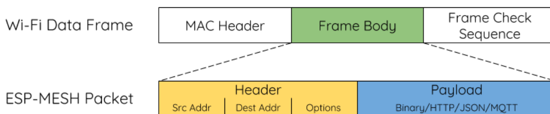
Fig. 54: ESP-WIFI-MESH Packet
