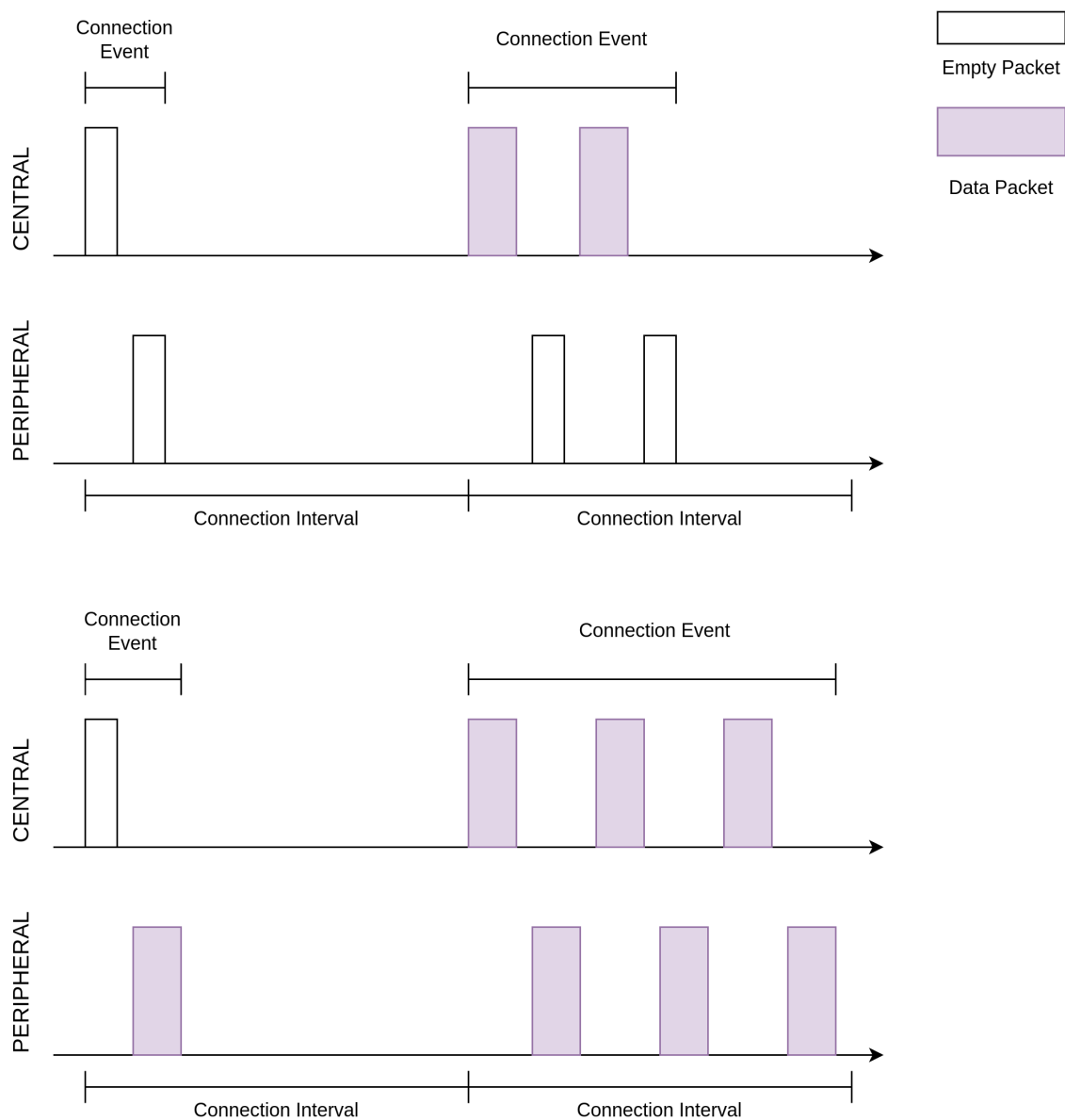
Fig. 20: 连接间隔与连接事件
