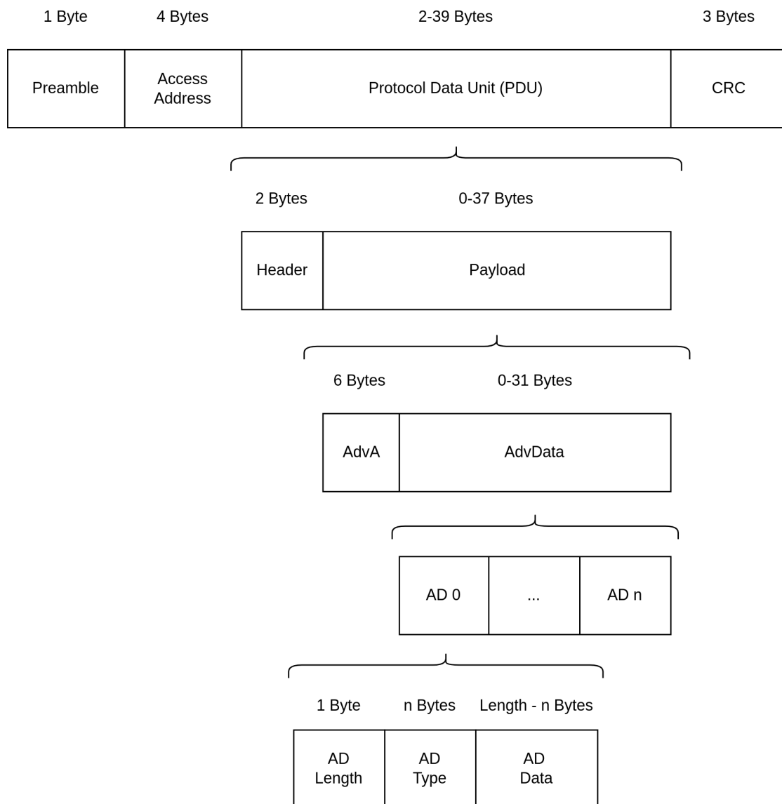
Fig. 14: Bluetooth LE 4.2 广播数据包结构
