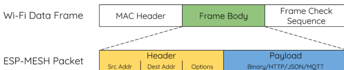
Fig. 57: ESP-WIFI-MESH Packet
