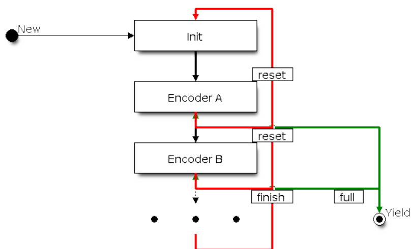
Fig. 14: RMT Encoder Chain
