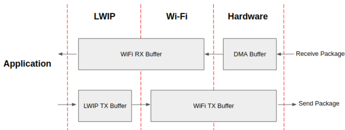
Fig. 63: ESP32-C6 datapath
