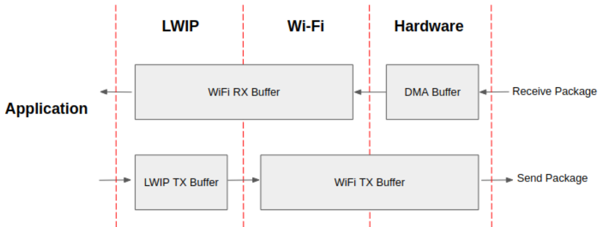
Fig. 64: ESP32-C6 datapath
