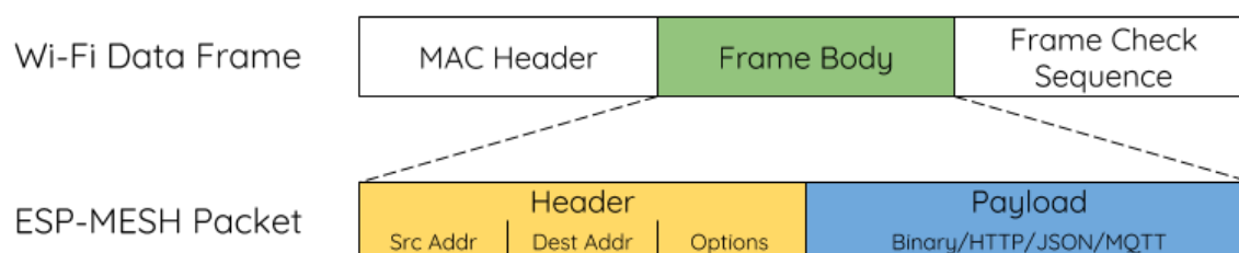
Fig. 36: ESP-WIFI-MESH Packet
