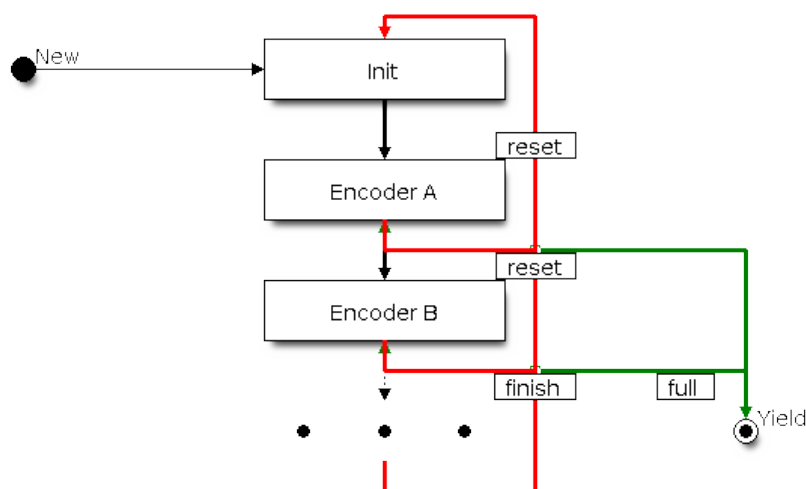
Fig. 18: RMT Encoder Chain
