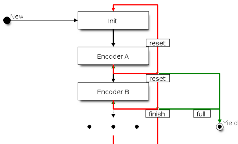
Fig. 16: RMT Encoder Chain
