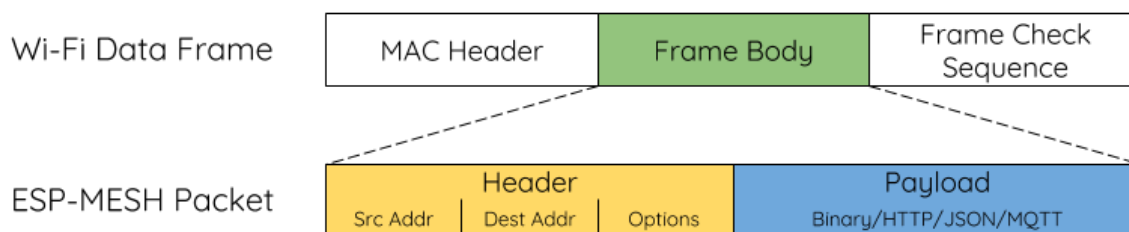
Fig. 59: ESP-WIFI-MESH Packet
