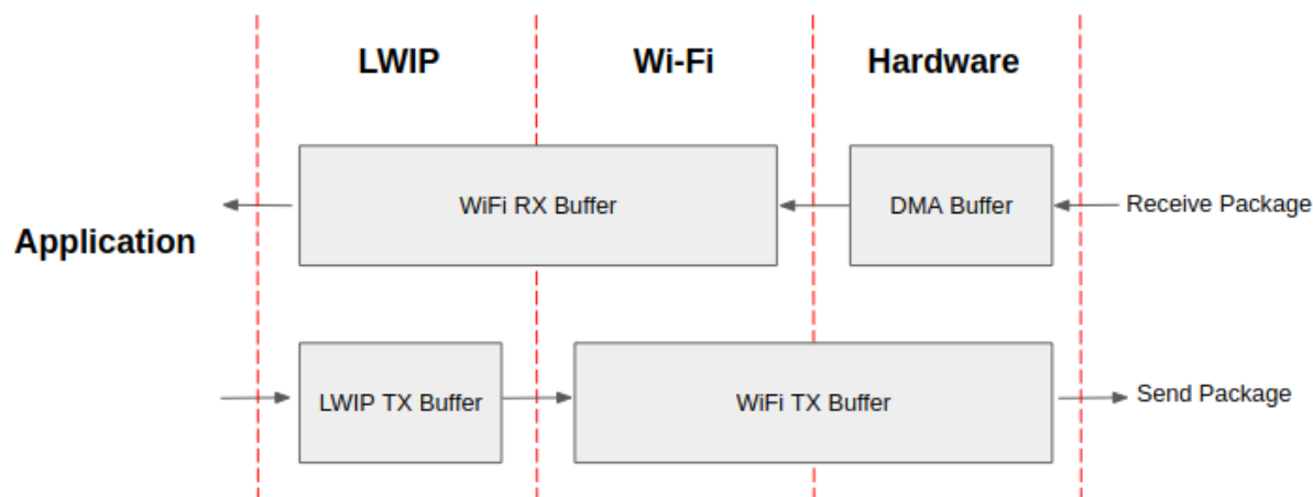
Fig. 67: ESP32-C6 datapath
