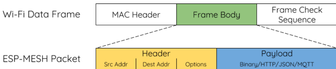
Fig. 59: ESP-WIFI-MESH Packet
