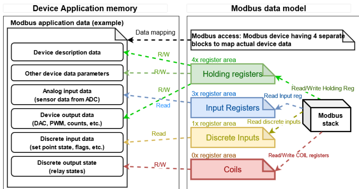
Fig. 18: Modbus data mapping
