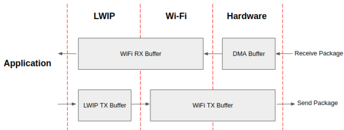
Fig. 33: ESP32-C2 datapath
