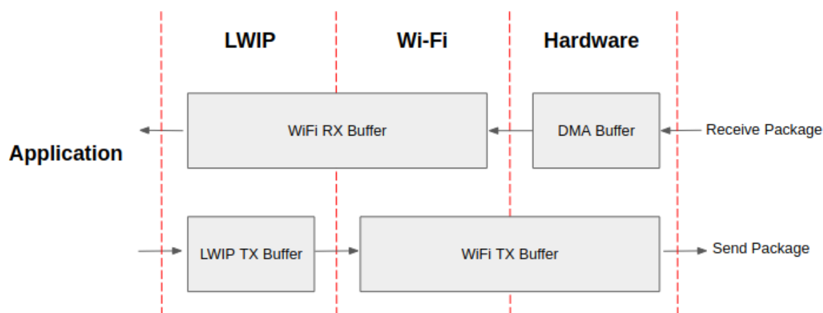
Fig. 33: ESP32-C2 datapath
