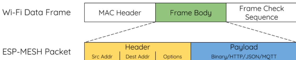
Fig. 37: ESP-WIFI-MESH Packet
