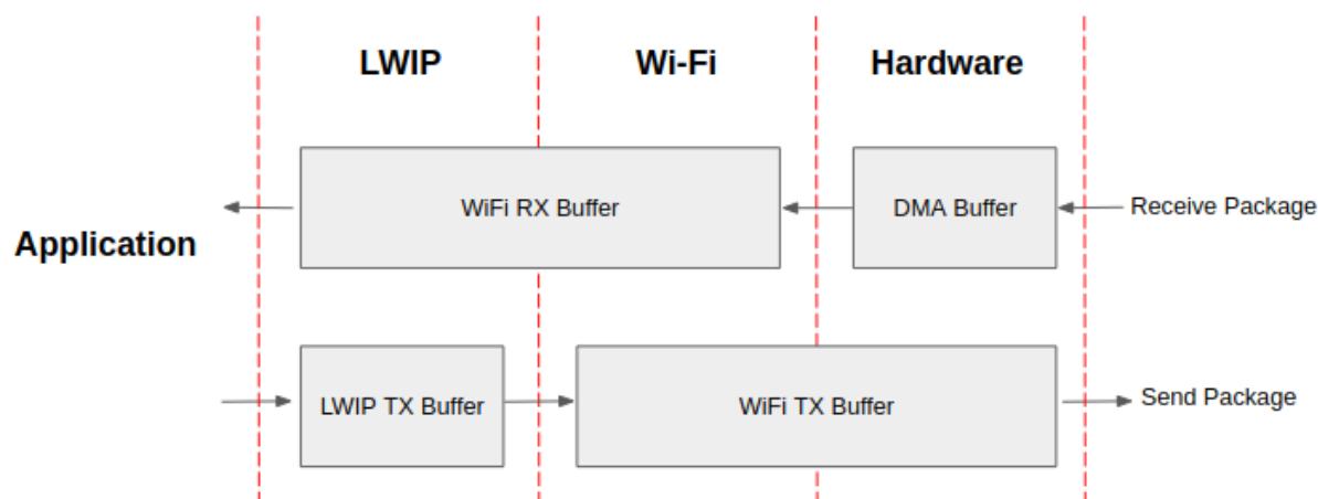
Fig. 64: ESP32-C6 datapath
