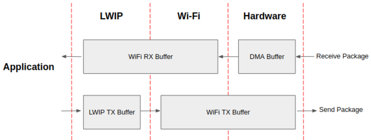
Fig. 37: ESP32-C2 datapath
