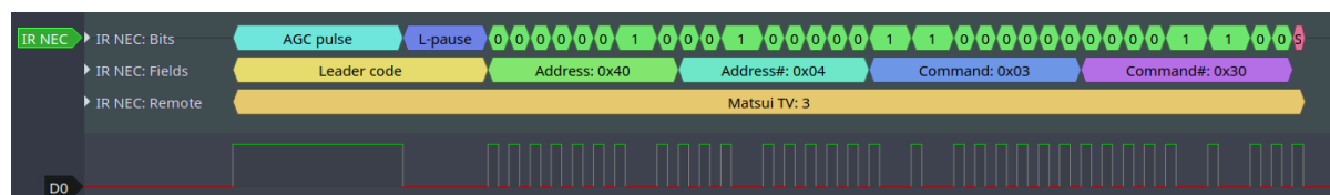
Fig. 23: IR NEC Frame
