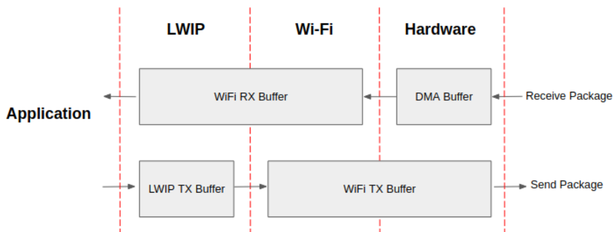
Fig. 67: ESP32-C6 datapath
