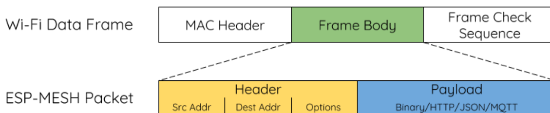
Fig. 60: ESP-WIFI-MESH Packet
