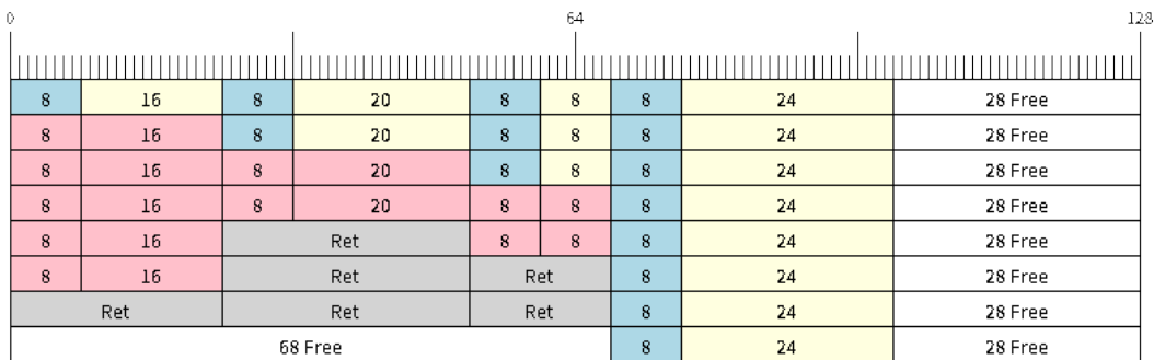
图 26: 在不可分割和可分割环形 buffer 中检索/返回数据项
