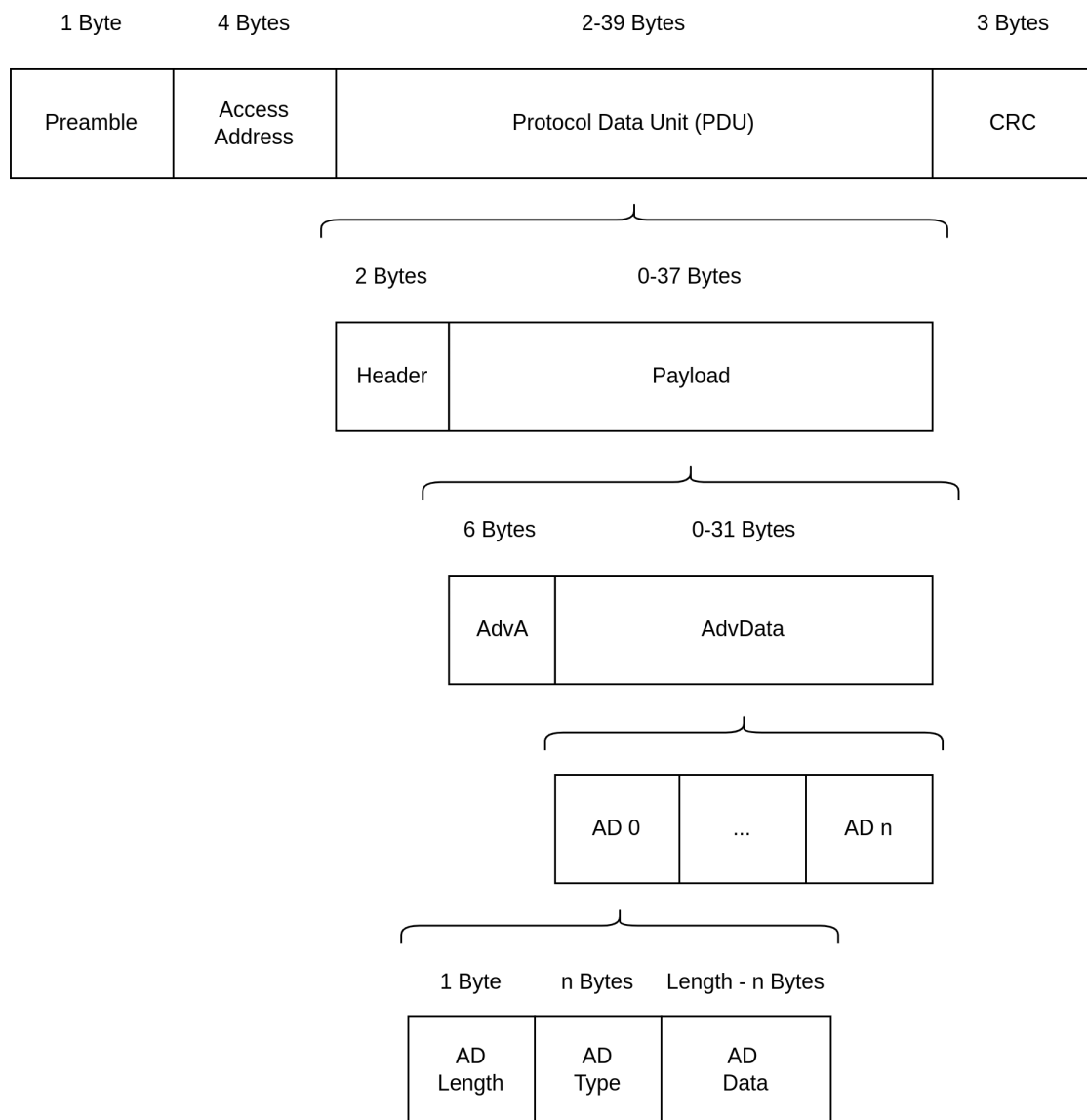
图 13: Bluetooth LE 4.2 广播数据包结构
