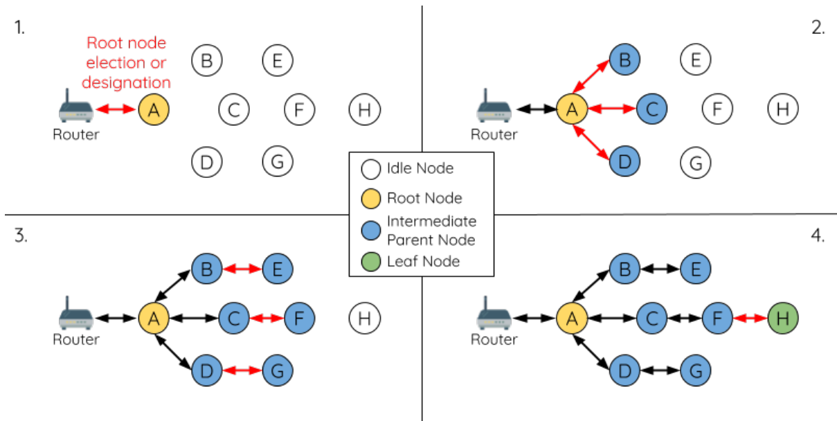
图 37: ESP-WIFI-MESH 网络构建过程
