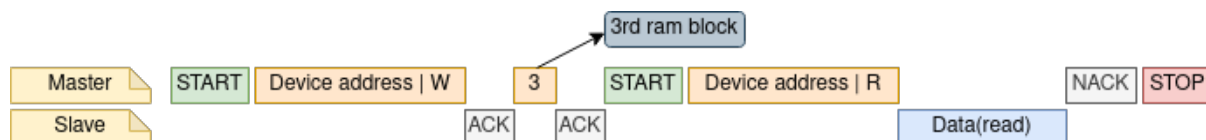
图 12: 从 I2C 从机 RAM 中获取数据
