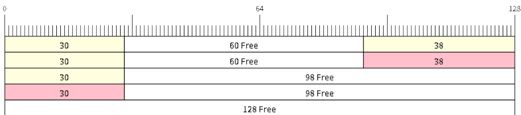
图 27: 在字节 buffer 中检索/返回数据
