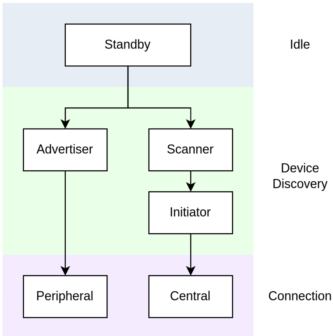
图 3: GAP 角色转换关系
