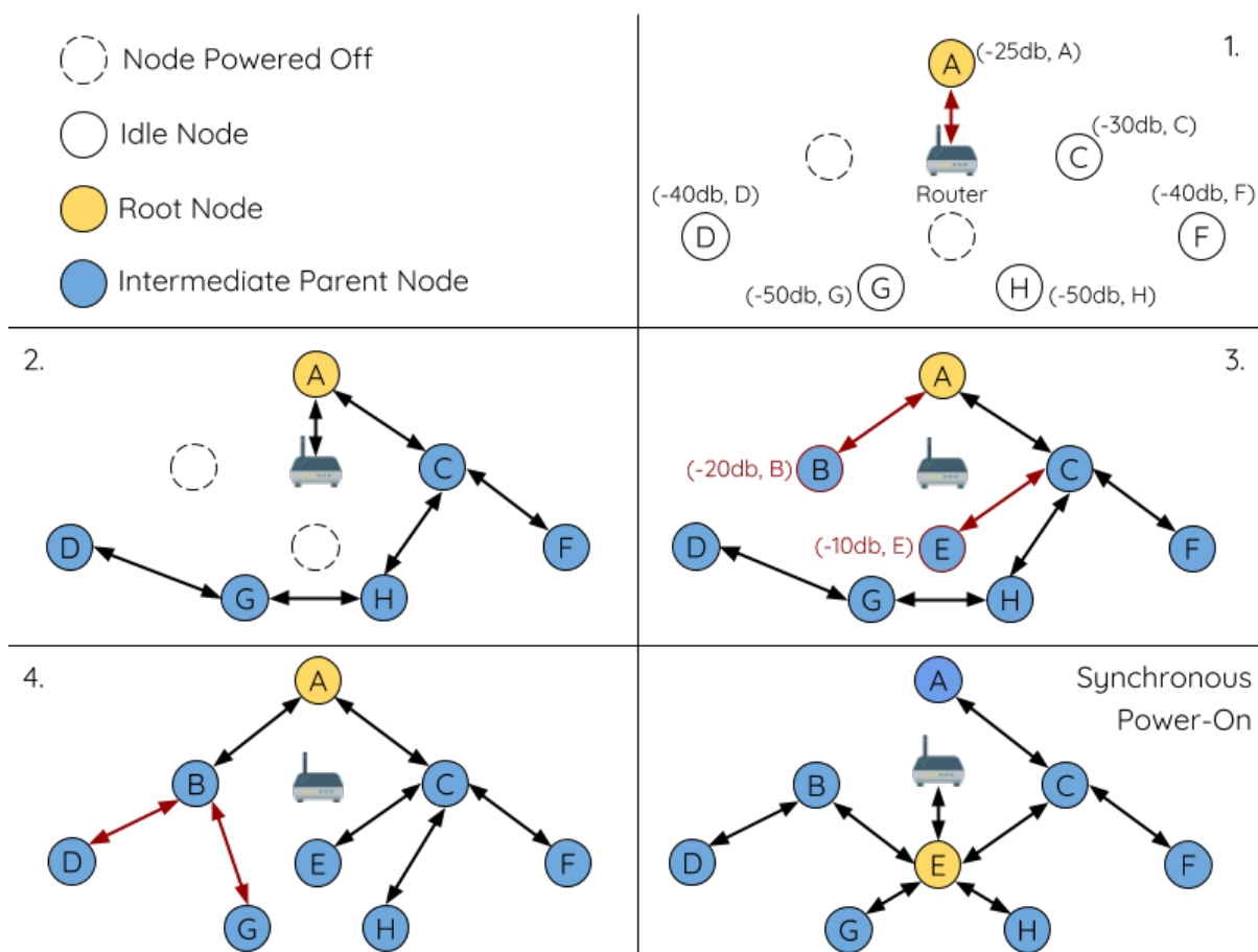
图 40: 网络构建 (异步电源) 示例
