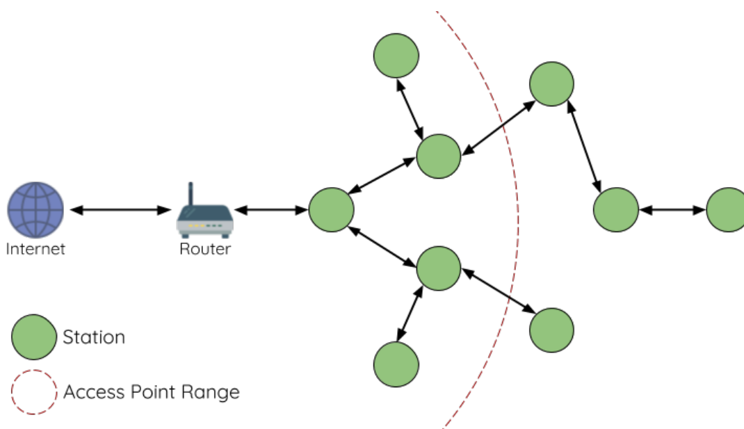
图 31: ESP-WIFI-MESH 网络架构示意图
