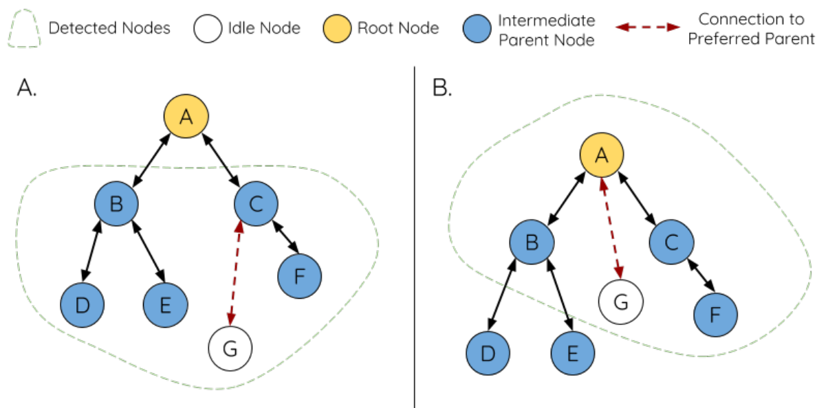
图 35: 首选父节点选择
