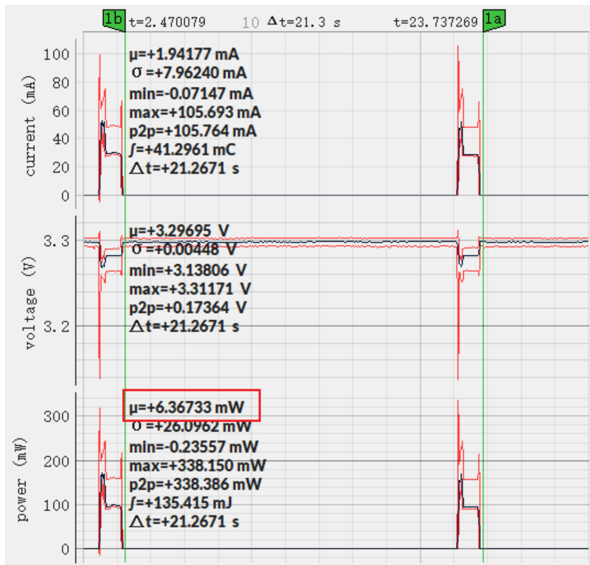
图 29: ESP32-S3-WROOM-1 的功耗 (点击放大)
