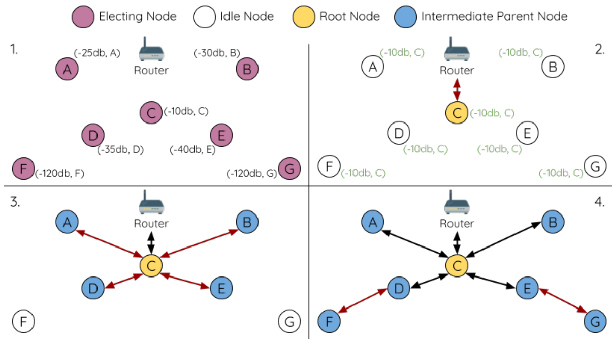
图 38: 根节点选举示例
