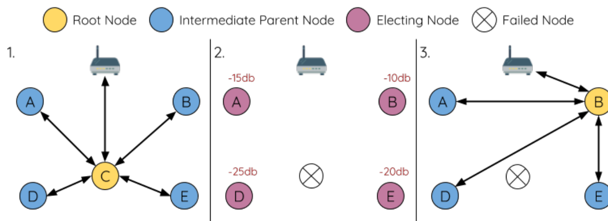
图 41: 根节点故障的自修复示意
