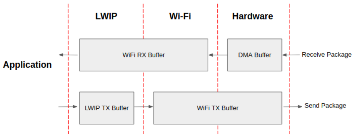
图 71: ESP32-C61 数据路径
