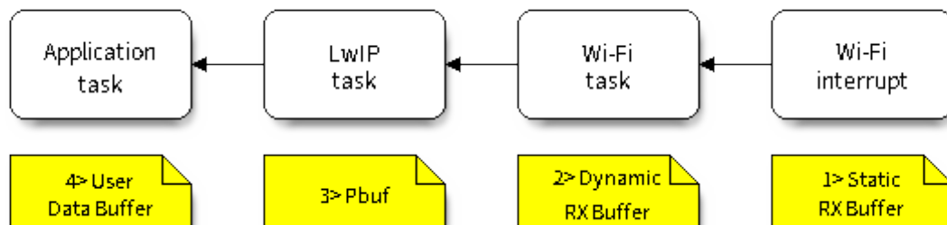
图 73: 接收数据缓冲区分配
