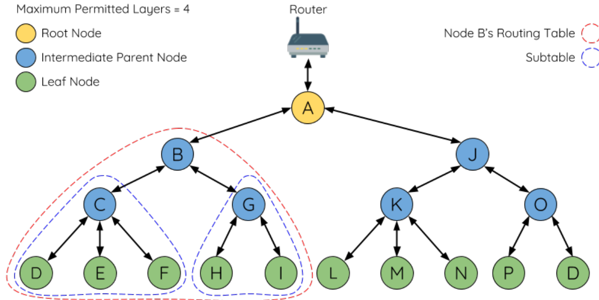
图 36: ESP-WIFI-MESH 路由表示例
