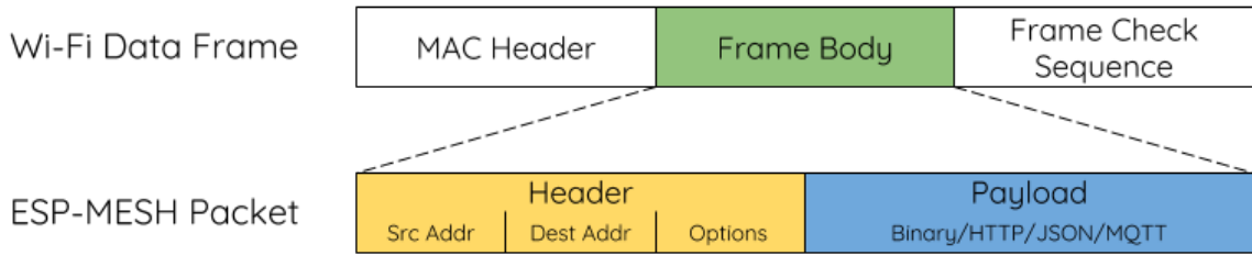
图 43: ESP-WIFI-MESH 数据包
