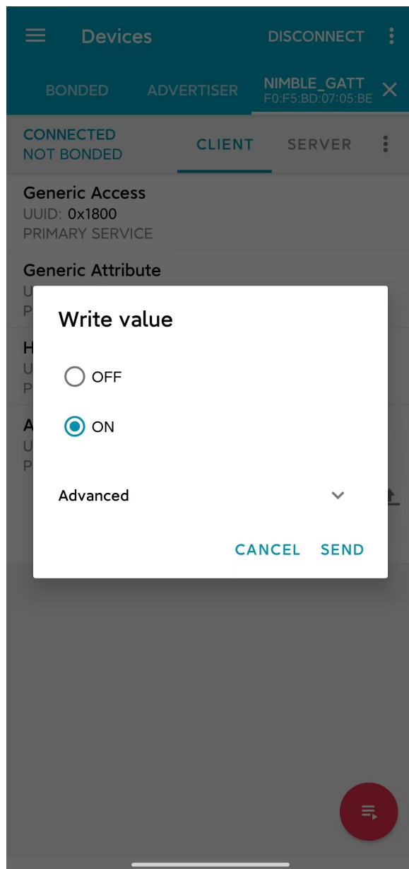
图 9: 对 LED 特征数据进行写访问
