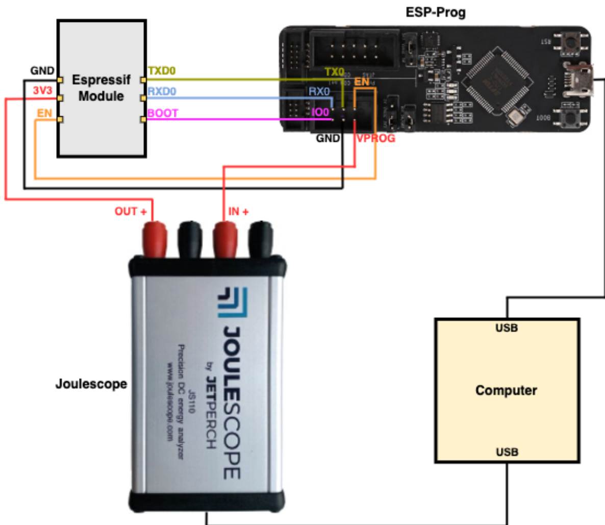
图 27: 硬件连接 (点击放大)
