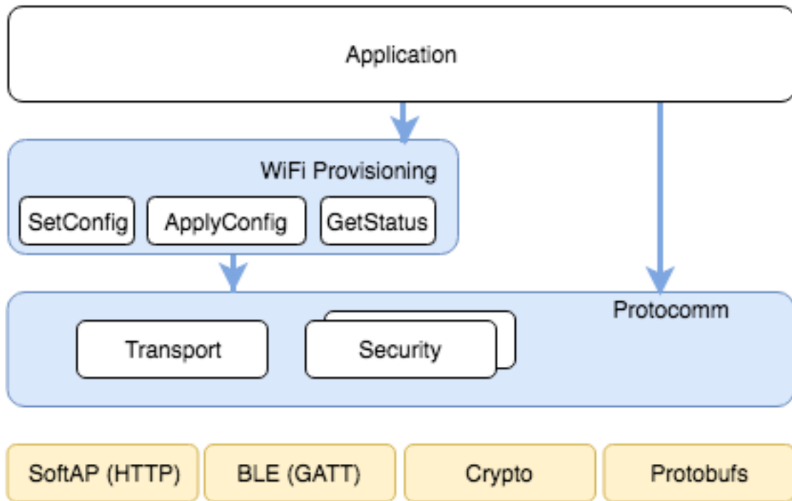
图 15: 统一配网架构
