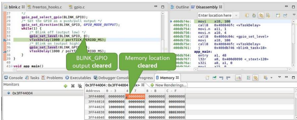
图 60: 观察内存地址 0x3FF44004 处的某个比特被置低
