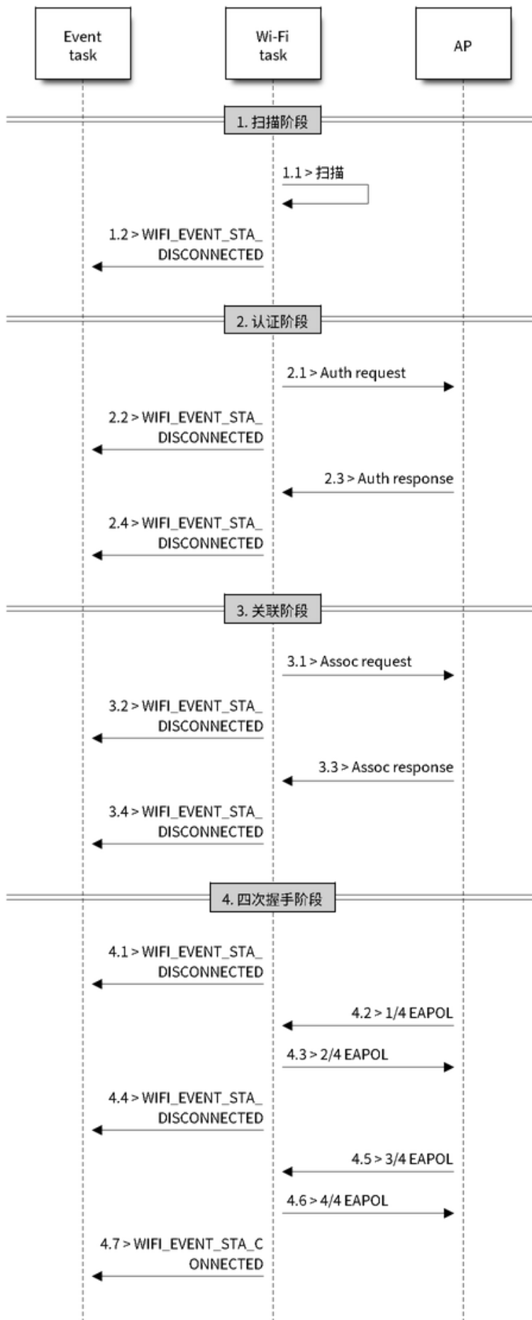
图 70: Wi-Fi station 连接过程
