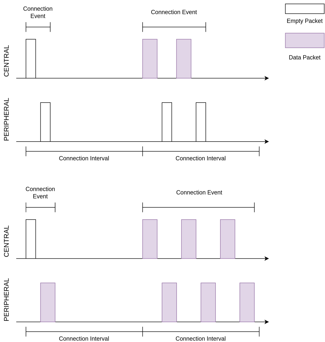
图 19: 连接间隔与连接事件
