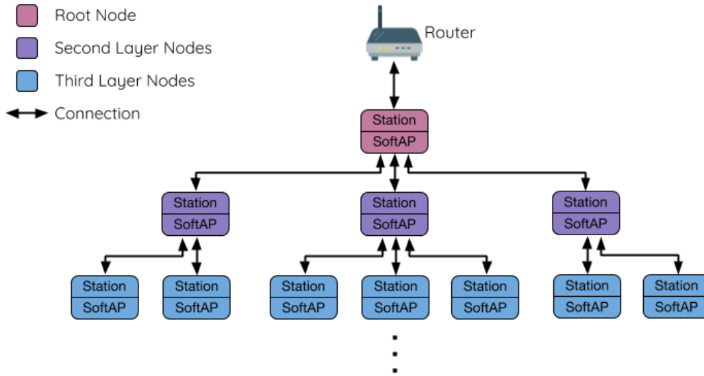
图 32: ESP-WIFI-MESH 树型拓扑
