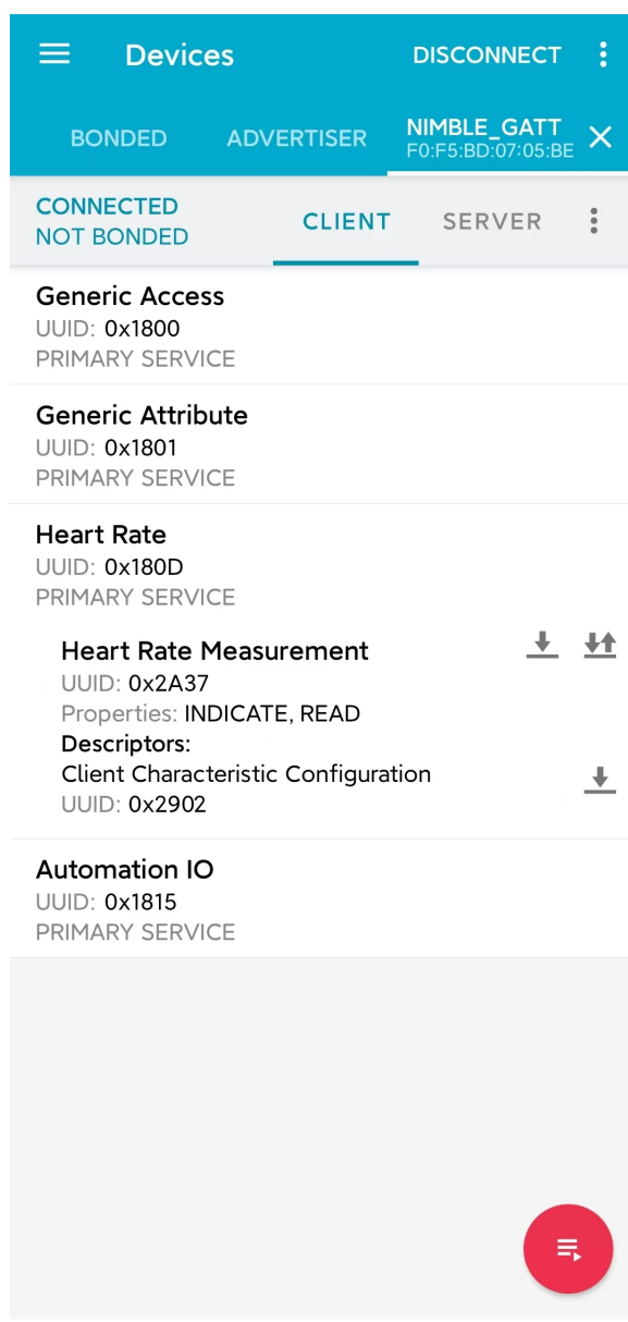
图 10: Heart Rate Service
