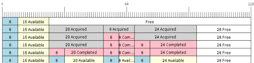
图 46: 在不可分割环形 buffer 中 SendAcquire/SendComplete 数据项
