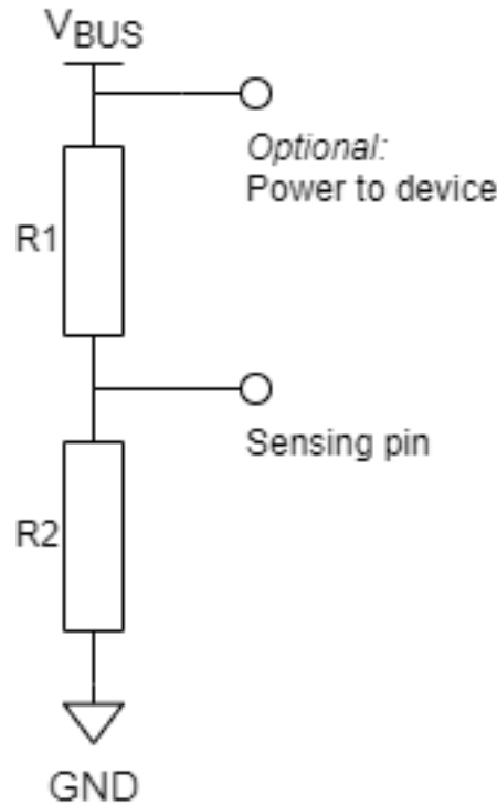
图 38: 用于 VBUS 监测的简易分压器
