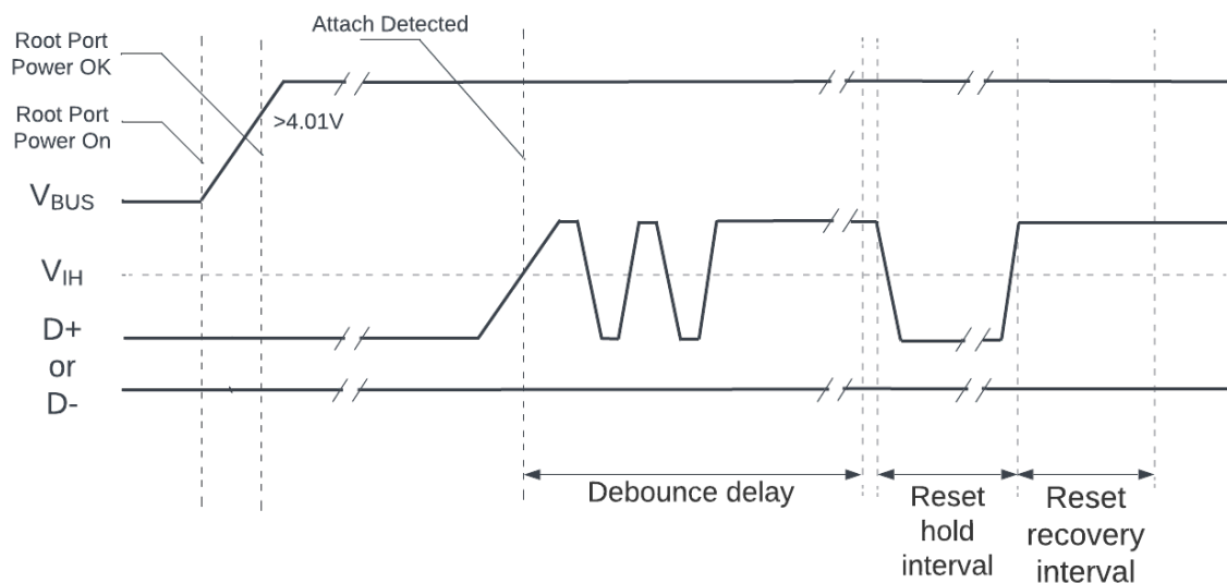
图 41: USB 根集线器上电和连接事件时序
