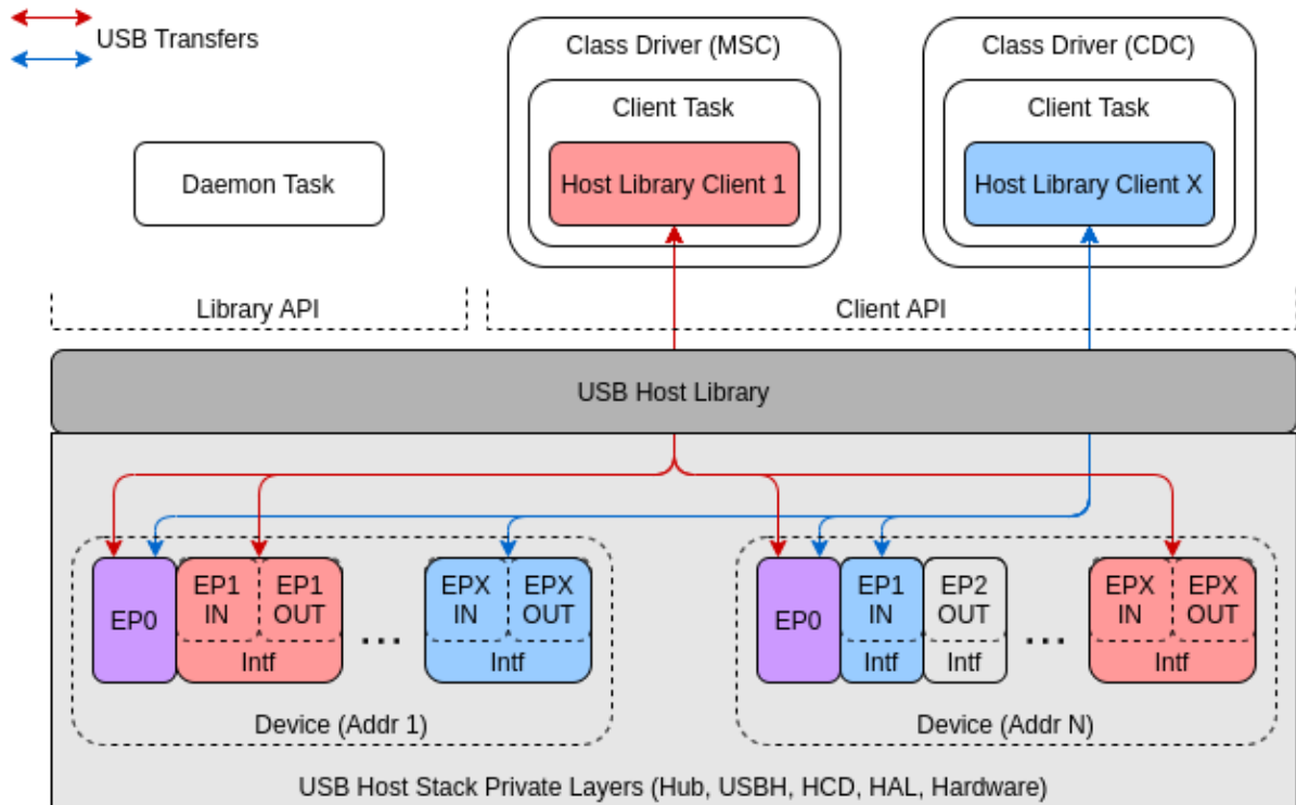
图 39: USB 主机功能涉及的关键实体
