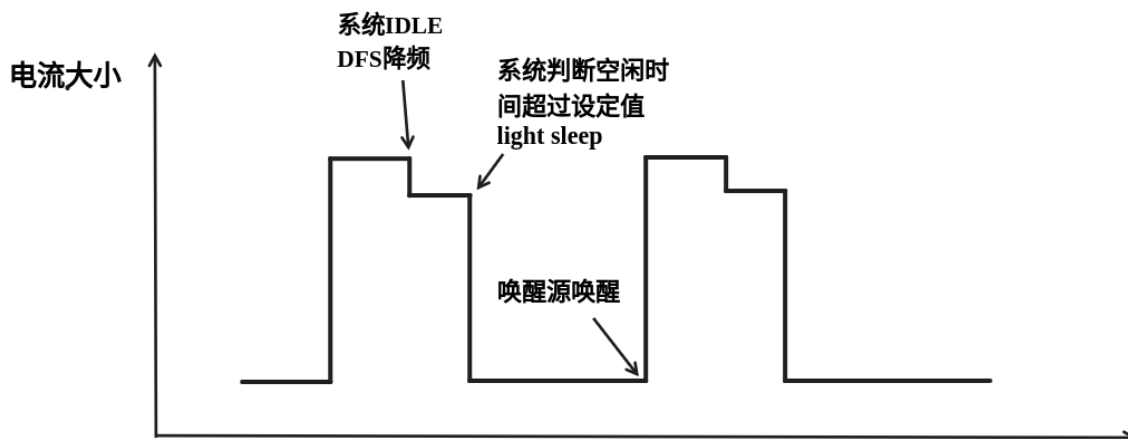
图 30: Auto Light-sleep 模式理想电流图
