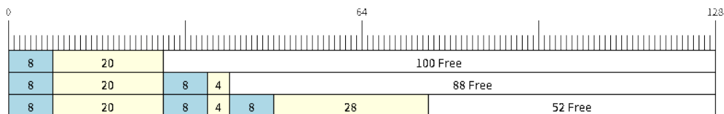
图 44: 向不可分割或可分割的环形 buffer 发送数据项
