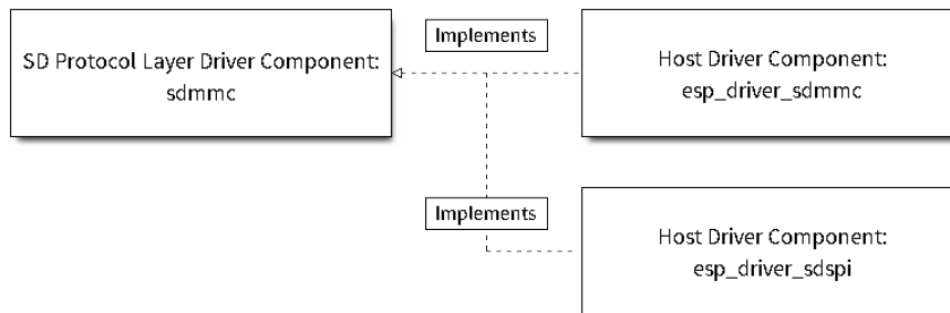
图 43: SD 主机端组件架构
