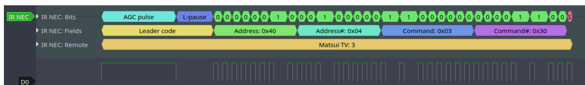
图 22: 红外 NEC 帧
