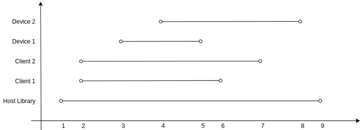
图 40: USB 主机库典型生命周期
