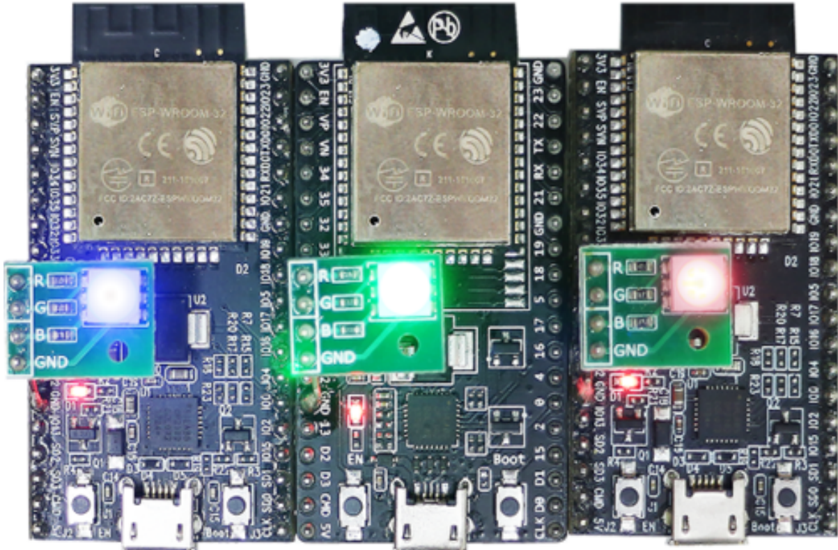
图 13: 3 个上电的 ESP-BLE-MESH 节点
