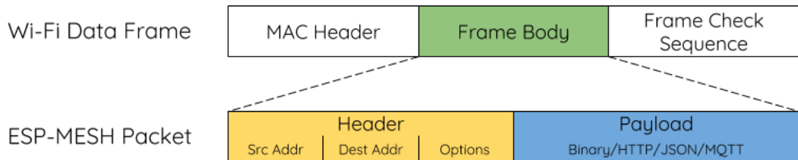
图 29: ESP-WIFI-MESH 数据包
