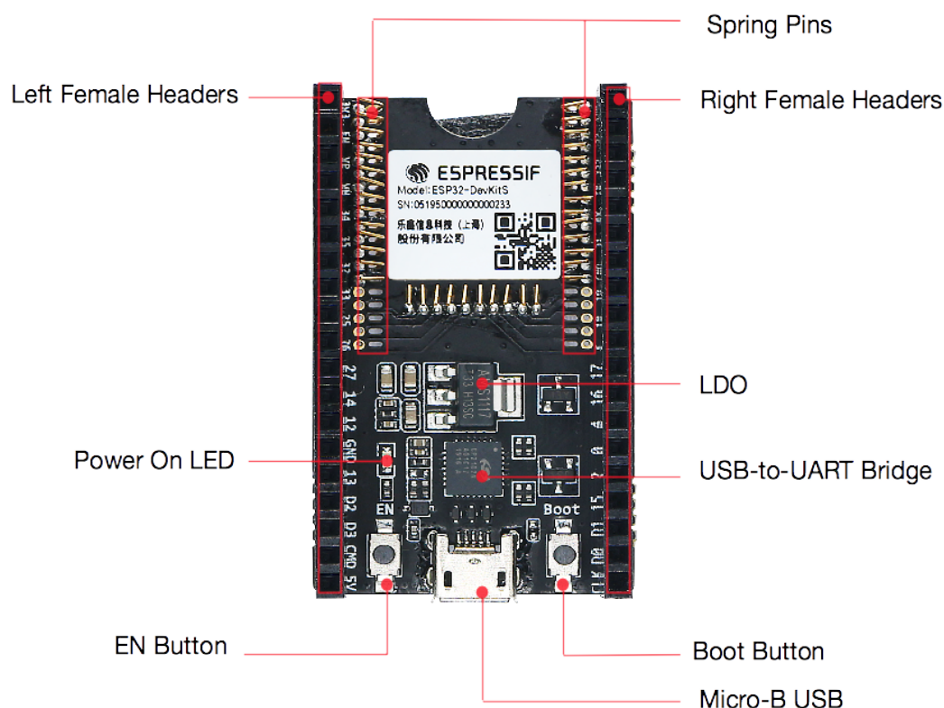
图 37: ESP32-DevKitS - 正面
