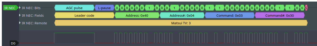
图 20: 红外 NEC 帧
