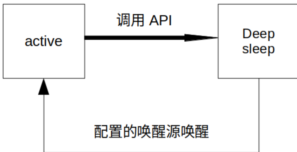
图 81: Deep-sleep 模式工作流程图
