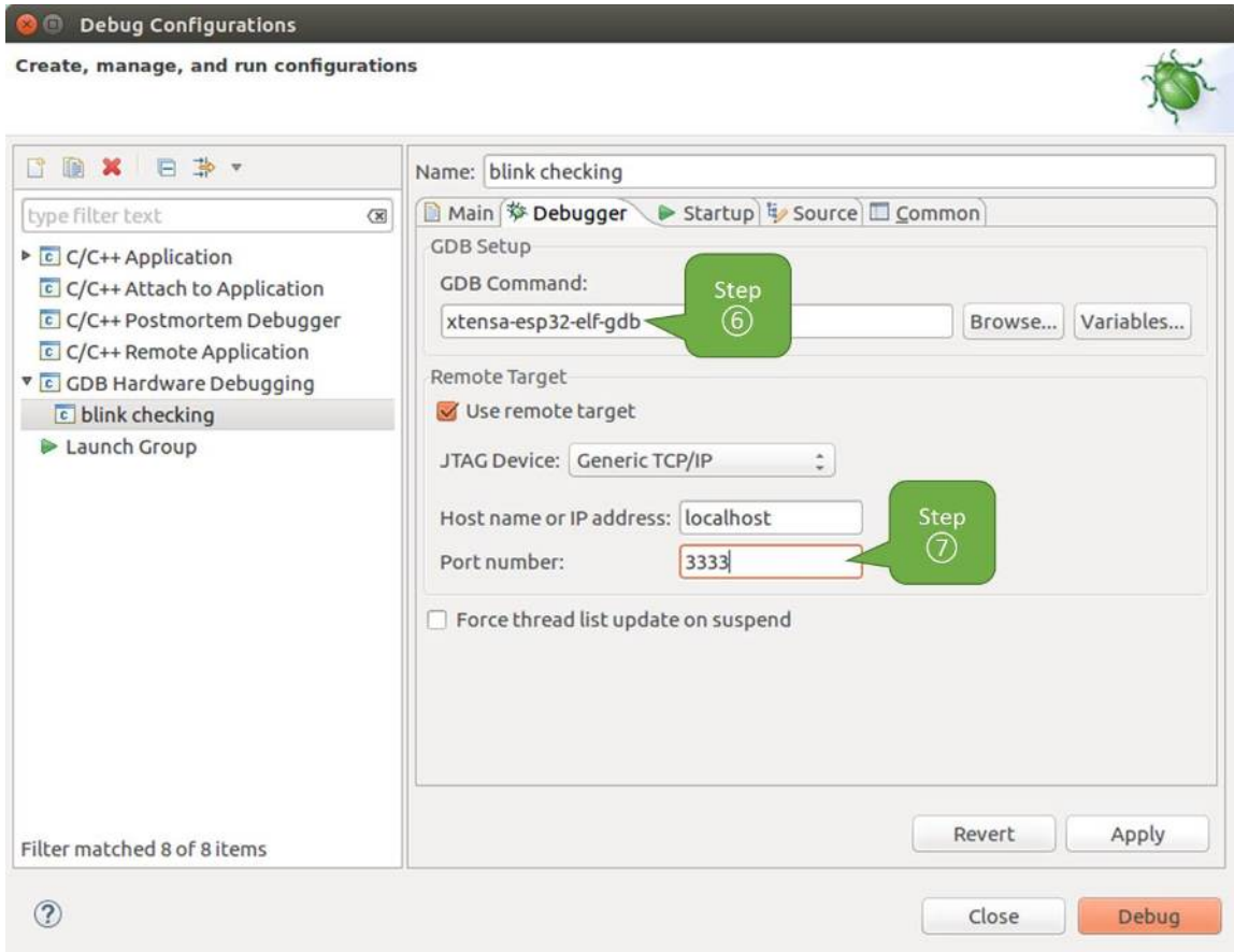
图 40: GDB 硬件调试的配置 - Debugger 选项卡
