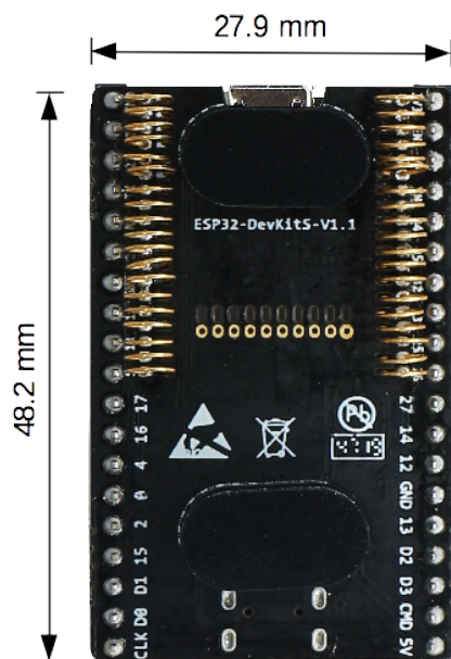
图 4: ESP32-DevKitS-R 尺寸 - 背面
