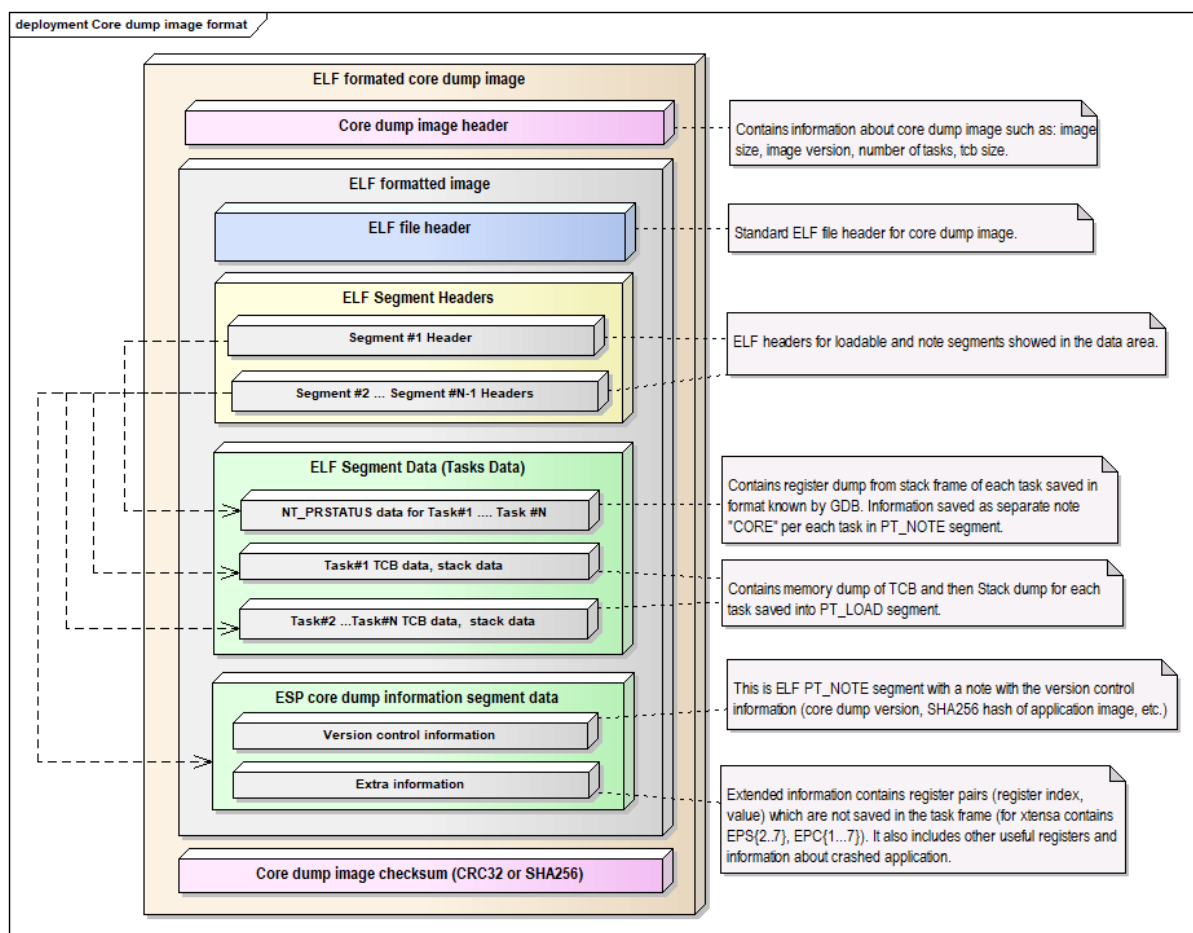
图 18: Core dump ELF image format
