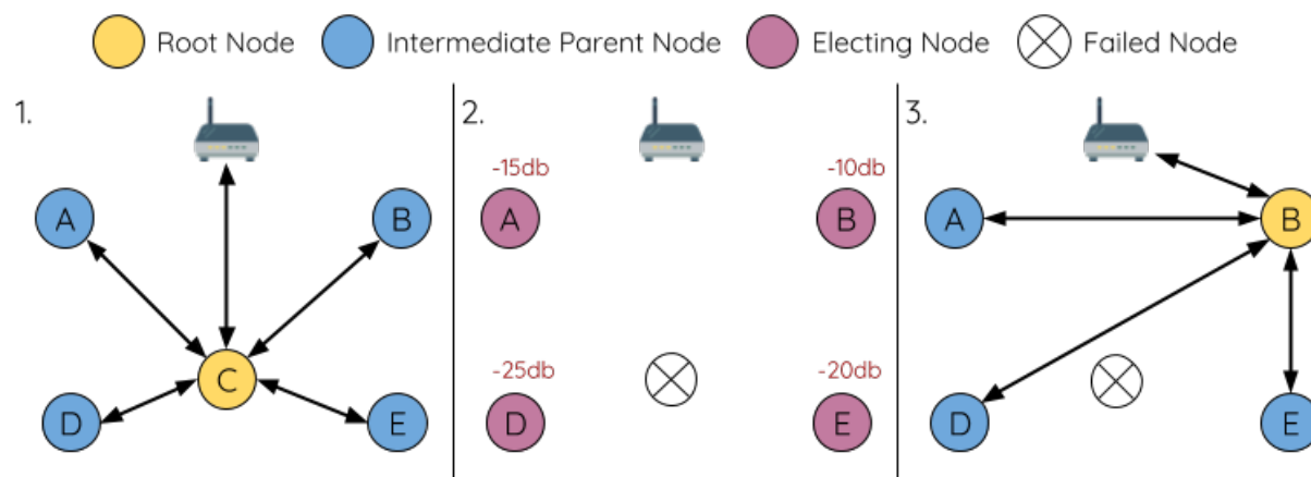
图 52: 根节点故障的自修复示意
